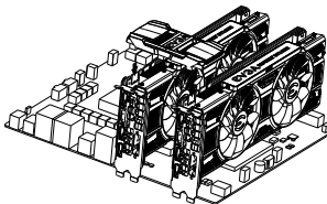
SLI de dos vías: Instale su segunda tarjeta GeForce en la ranura PCI Express x16 secundaria. Conecte las dos tarjetas usando el nuevo puente SLI de 2 vías que viene con su motherboard compatible con SLI.
