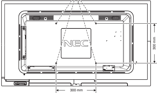
Interfaz de montaje VESA (M6)
