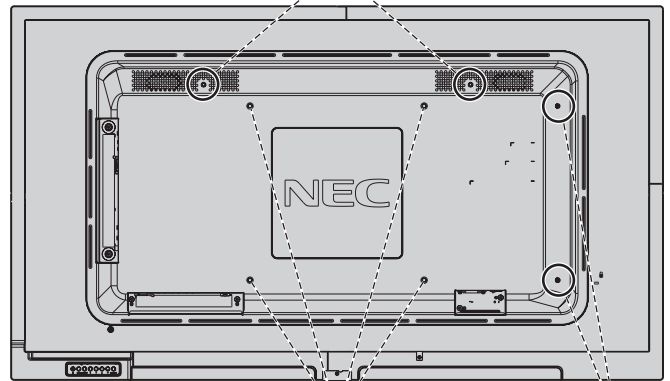
Interfaz de montaje VESA (M6)
