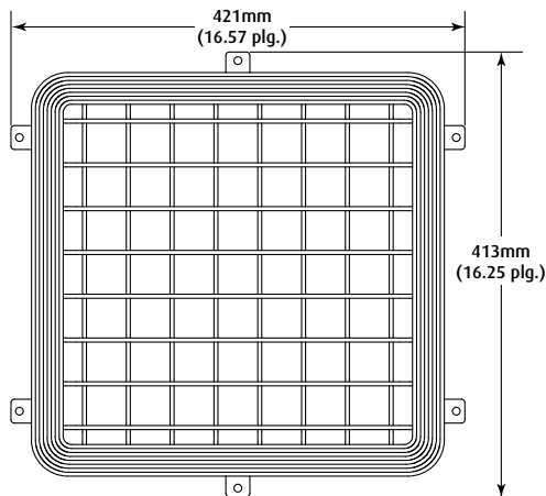
DIMENSIONES EXTERIORES
