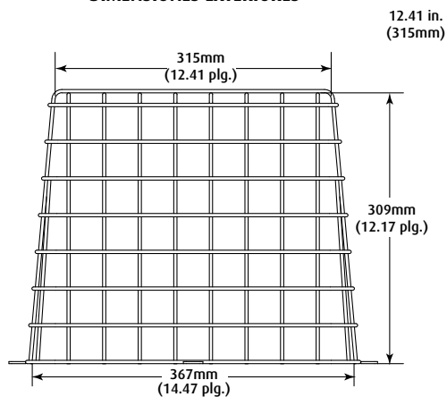
DIMENSIONES INTERIORES
