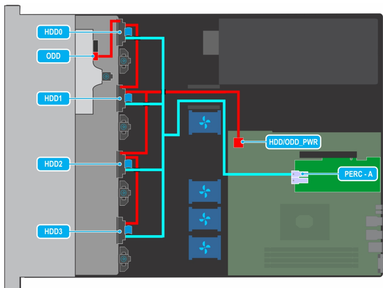
Figura 65. Colocación de los cables: unidad cableada de 4 x 3.5 pulgadas con PERC
