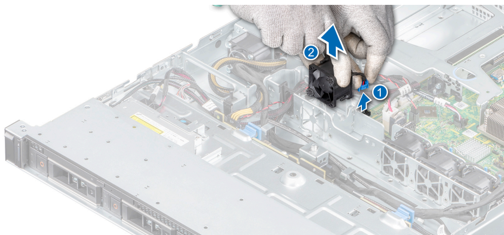
Figura 17. Extracción de un ventilador de refrigeración
