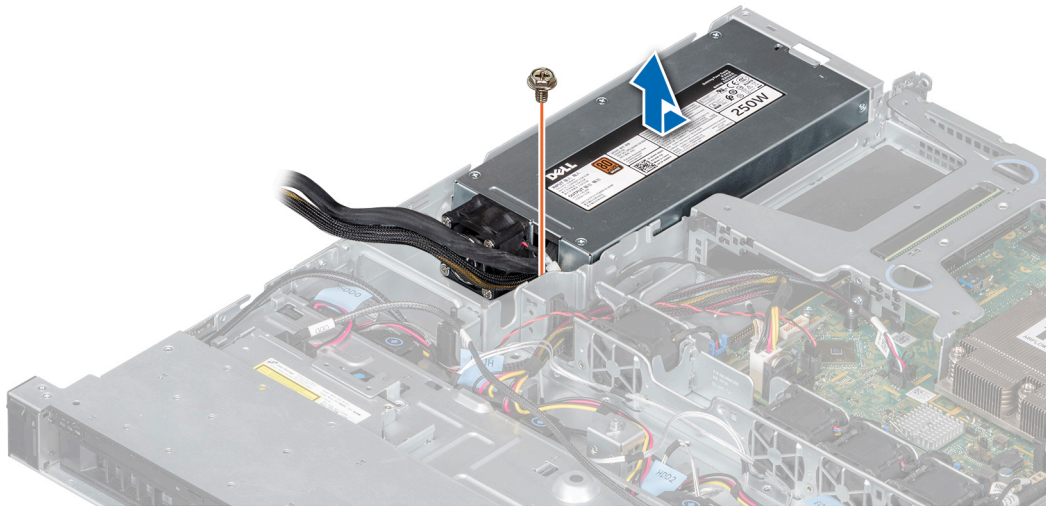
Figura 69. Extracción de una unidad de fuente de alimentación cableada
