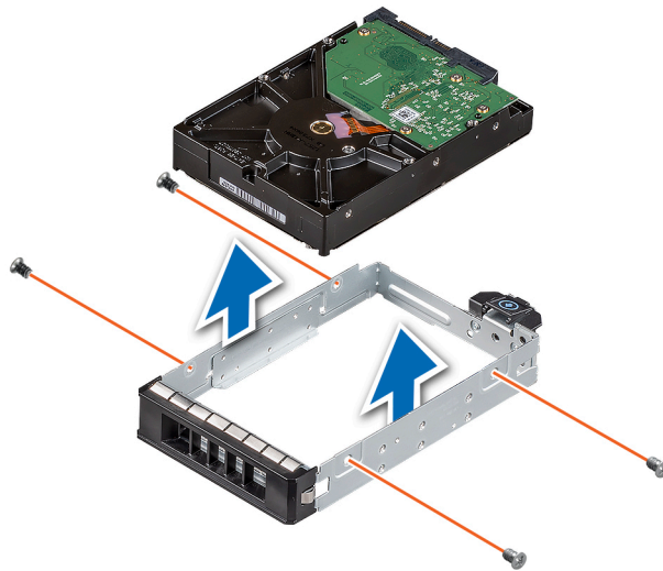
Figura 31. Extracción de la unidad cableada del portaunidades
