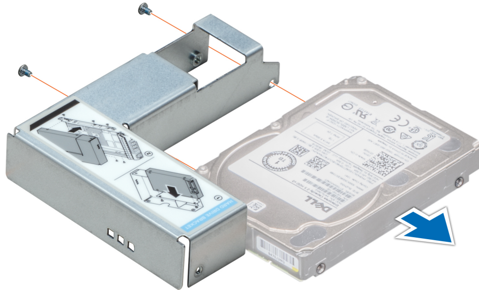
Figura 25. Extracción de una unidad de 2.5 pulgadas de un adaptador de unidad de 3.5 pulgadas
