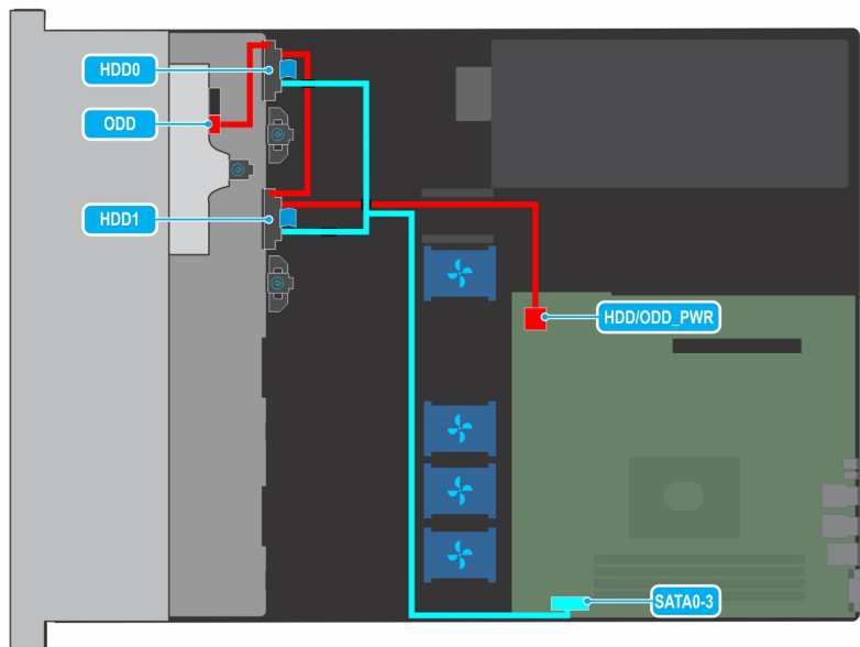
Figura 68. Colocación de los cables: unidad cableada de 2 x 3.5 pulgadas con SATA
