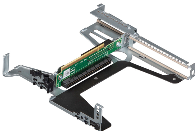
Figura 38. Soporte vertical para tarjetas de expansión
