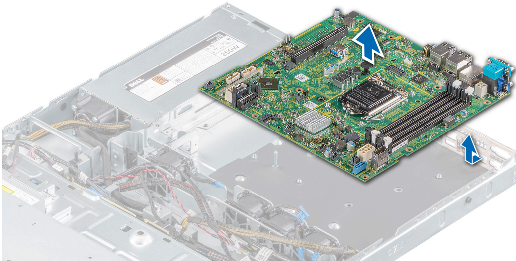
Figura 72. Extracción de la placa base
