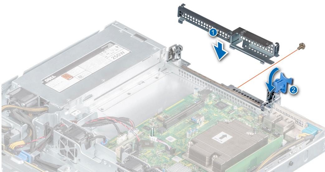
Figura 40. Instalación del soporte vertical para tarjetas de expansión de relleno
