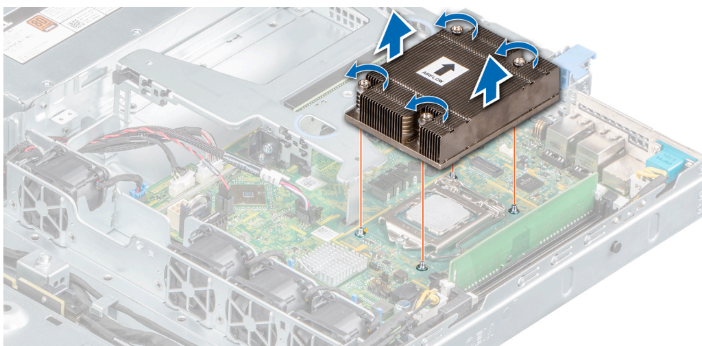
Figura 53. Extracción del disipador de calor
