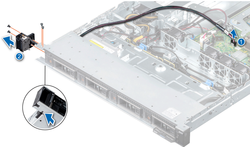
Figura 75. Extracción del panel de control izquierdo
