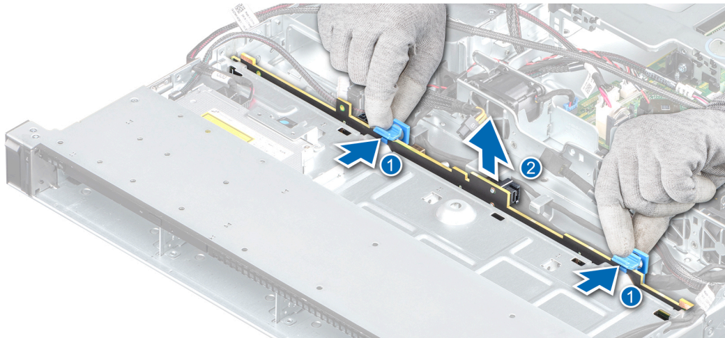
Figura 61. Extracción del backplane de unidad
