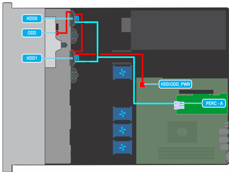
Figura 67. Colocación de los cables: unidad cableada de 2 x 3.5 pulgadas con PERC
