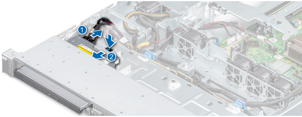
Figura 51. Extracción de la unidad óptica opcional
