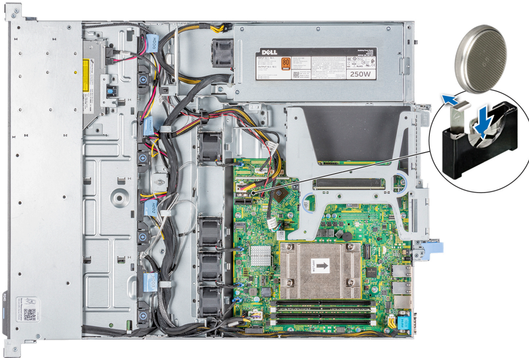
Figura 50. Instalación de la batería del sistema
