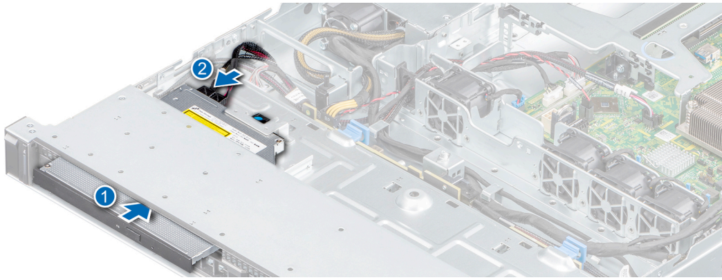
Figura 52. Instalación de la unidad óptica opcional
