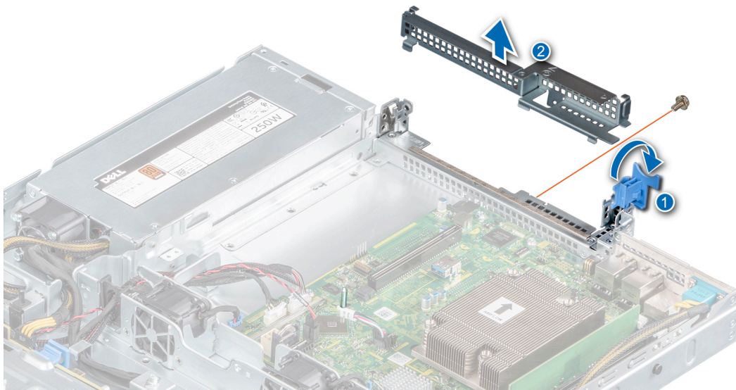
Figura 41. Extracción del soporte vertical para tarjetas de expansión de relleno
