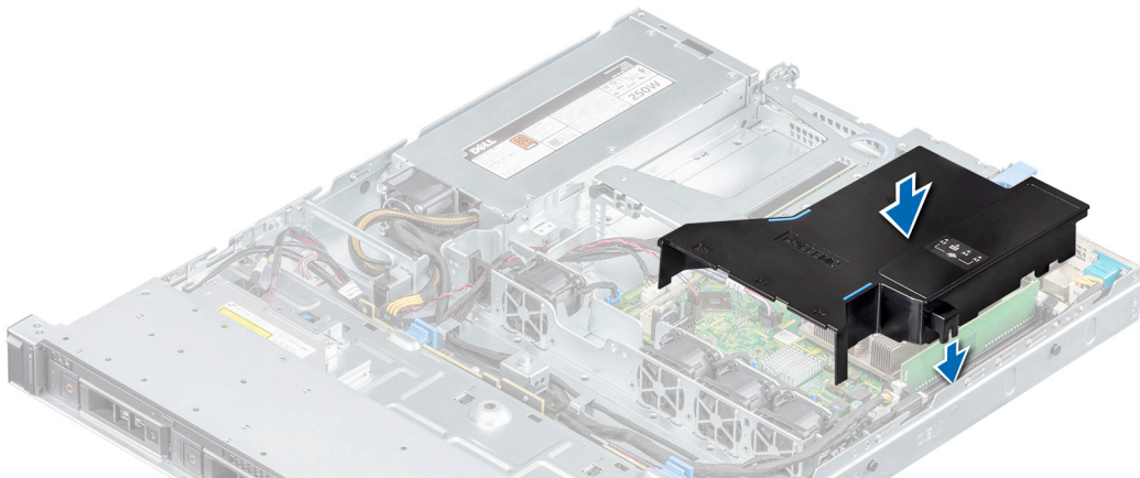
Figura 14. Instalación de la cubierta para flujo de aire
