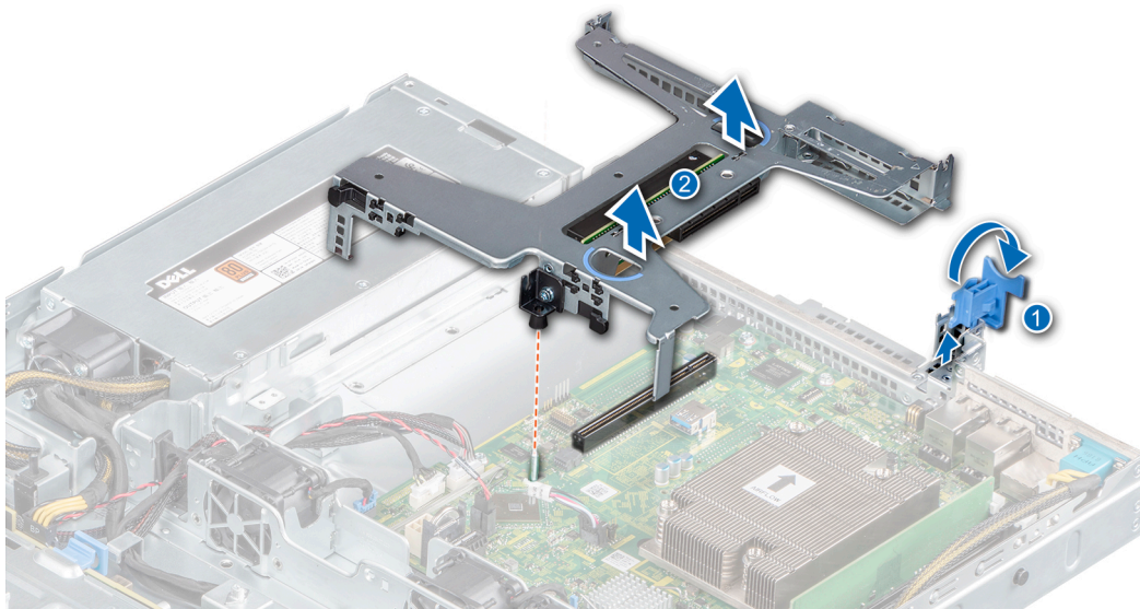
Figura 39. Extracción del soporte vertical de tarjetas de expansión
