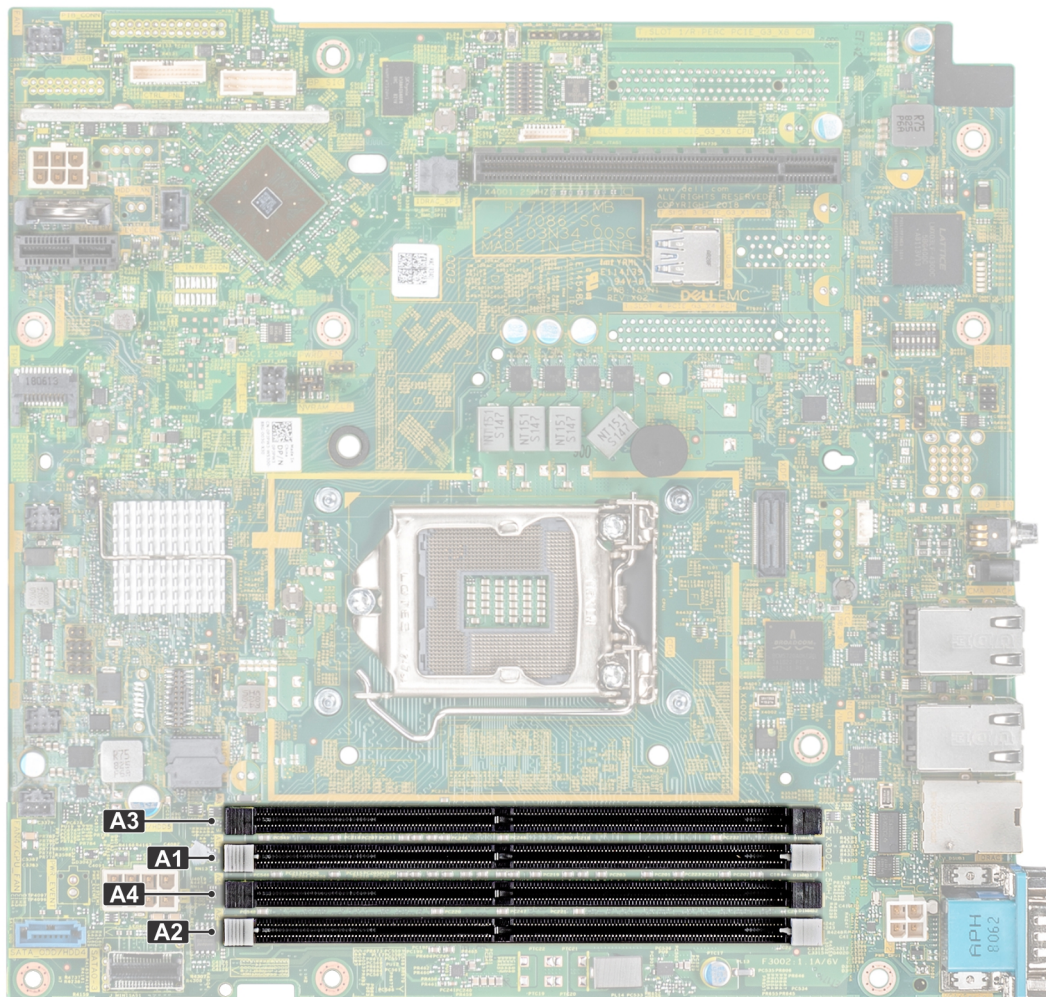
Figura 35. Ubicaciones de los sockets de memoria
