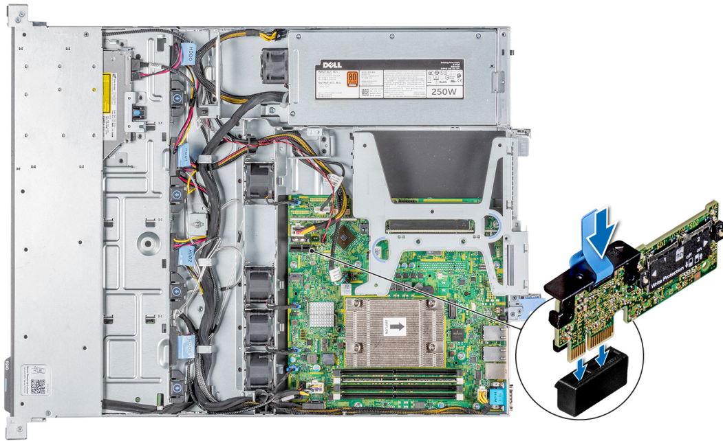
Figura 57. Instalación de la tarjeta vFlash o IDSDM opcional
