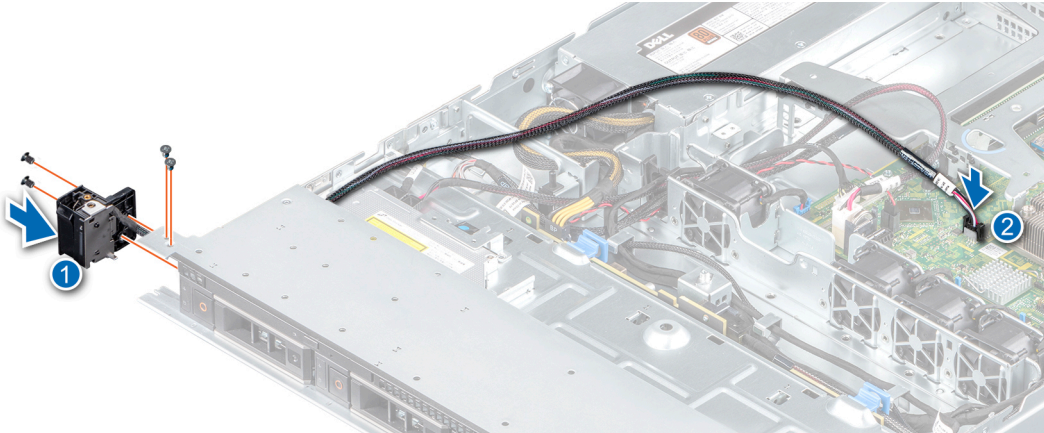
Figura 76. Instalación del panel de control izquierdo
