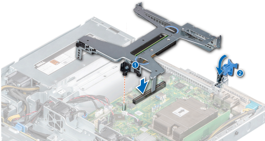
Figura 42. Instalación del soporte vertical de tarjetas de expansión
