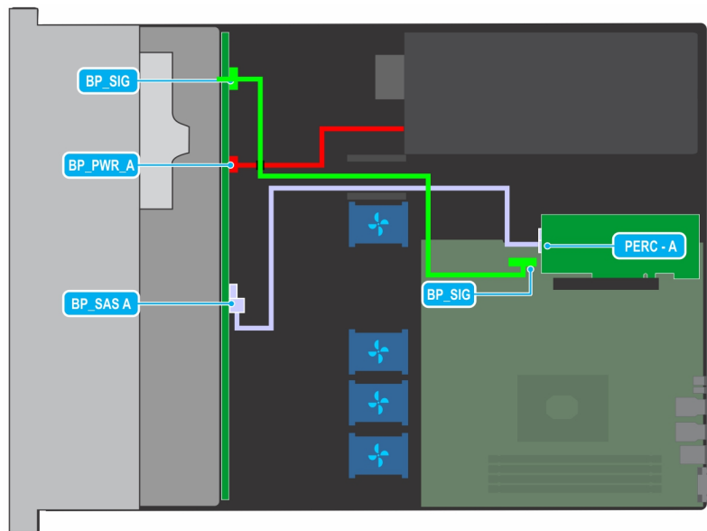
Figura 63. Colocación de los cables: backplane de unidad de 4 x 3.5 pulgadas con PERC
