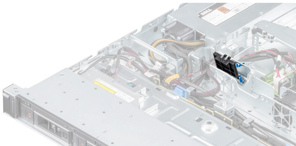
Figura 16. Instalación del ventilador de relleno
