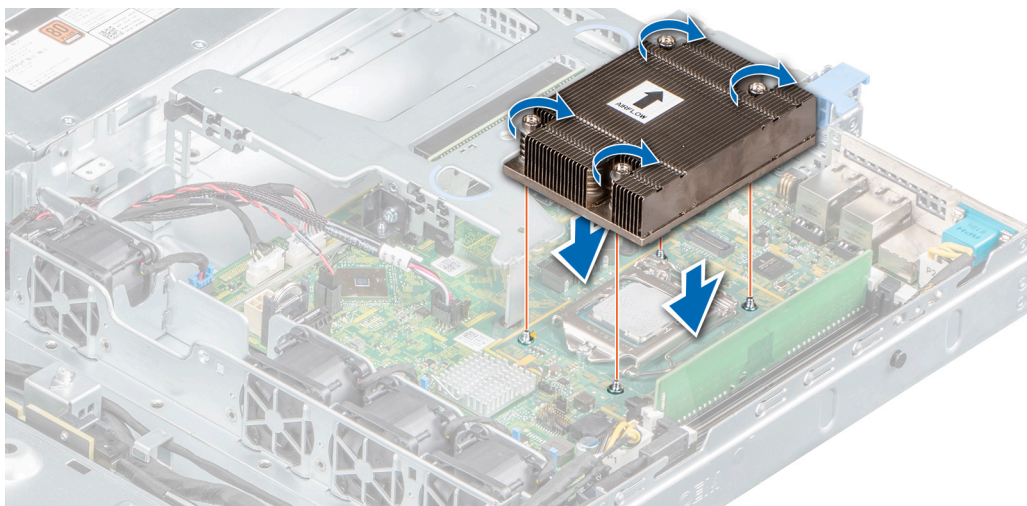
Figura 56. Instalación del disipador de calor
