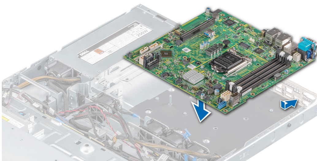
Figura 73. Instalación de la placa base
