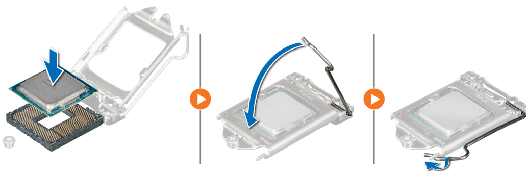
Figura 55. Instalación del procesador
