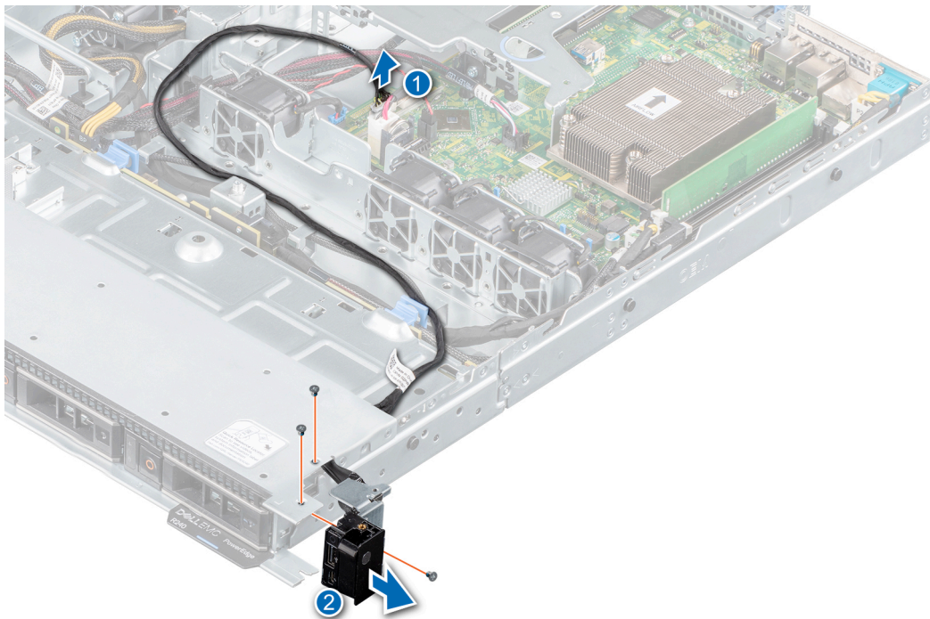
Figura 77. Extracción del panel de control derecho
