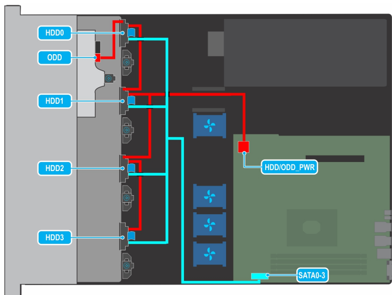
Figura 66. Colocación de los cables: unidad cableada de 4 x 3.5 pulgadas con SATA
