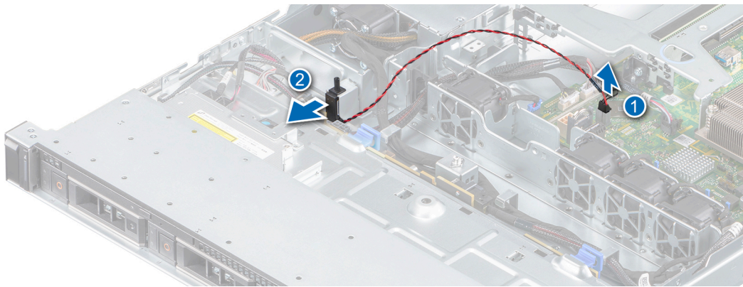
Figura 33. Extracción del interruptor de intrusiones
