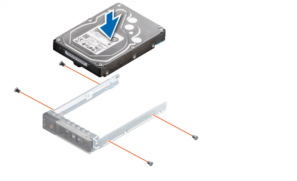
Figura 24. Instalación de una unidad en el portaunidades
