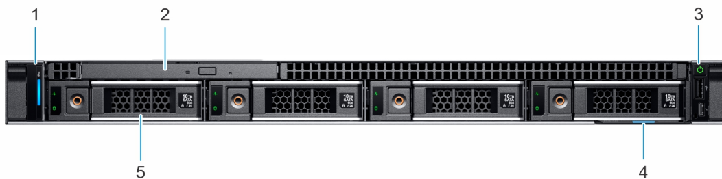
Figura 1. Vista frontal del sistema de unidad de 4 x 3.5 pulgadas
