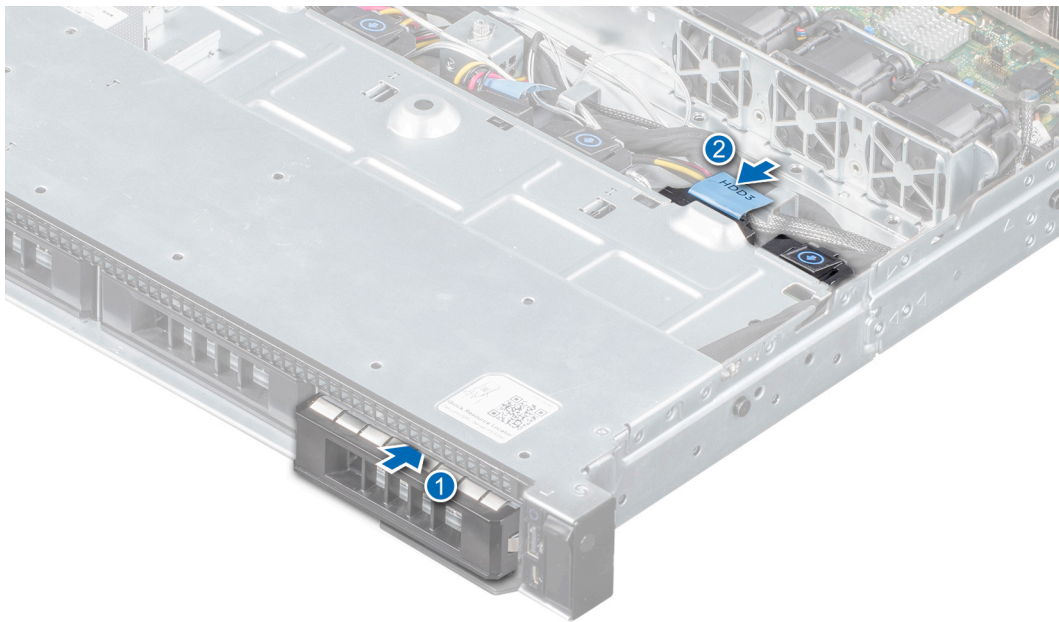
Figura 30. Instalación de una unidad cableada
