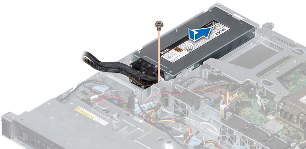
Figura 70. Instalación de una unidad de fuente de alimentación cableada
