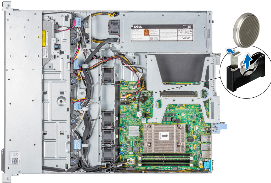
Figura 49. Extracción de la batería del sistema
