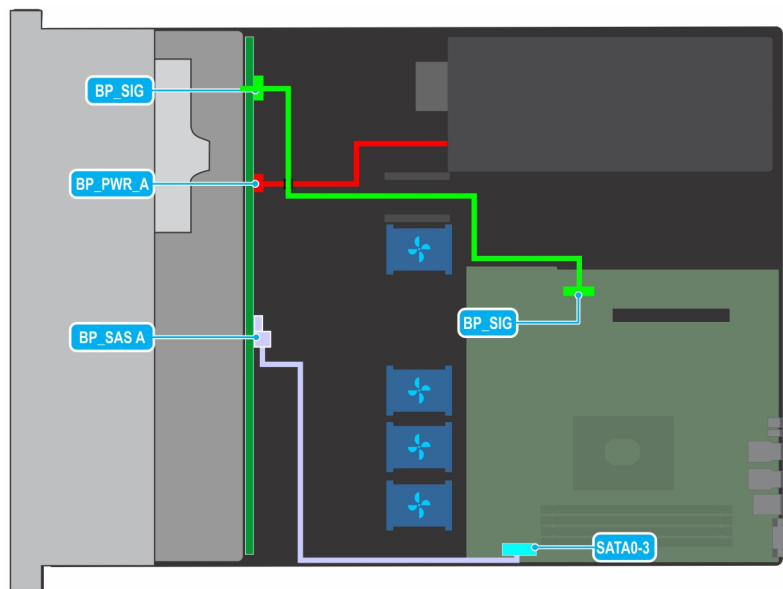
Figura 64. Colocación de los cables: backplane de unidad de 4 x 3.5 pulgadas con SATA
