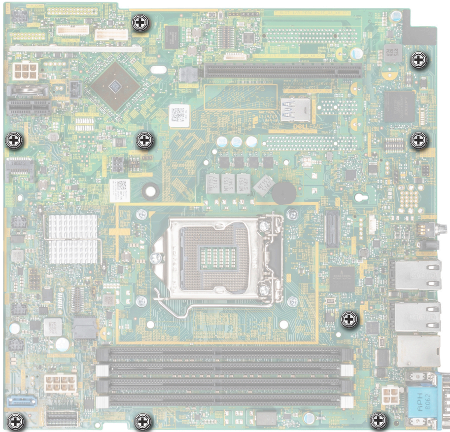
Figura 71. Tornillos que fijan la tarjeta madre del sistema
