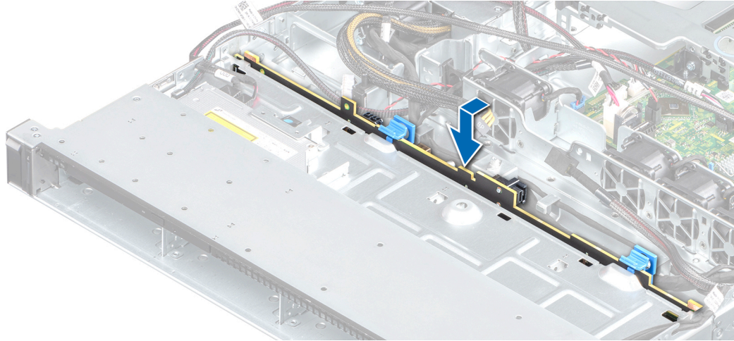
Figura 62. Instalación del plano posterior
