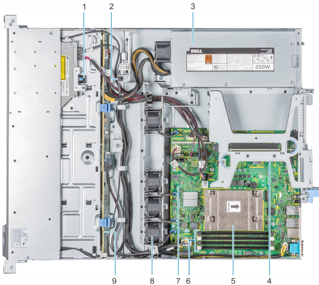
Figura 6. Interior del sistema: sistema de unidad de 4 x 3.5 pulgadas
