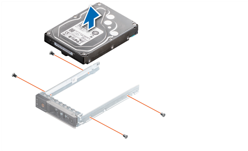
Figura 23. Extracción de una unidad del portaunidades
