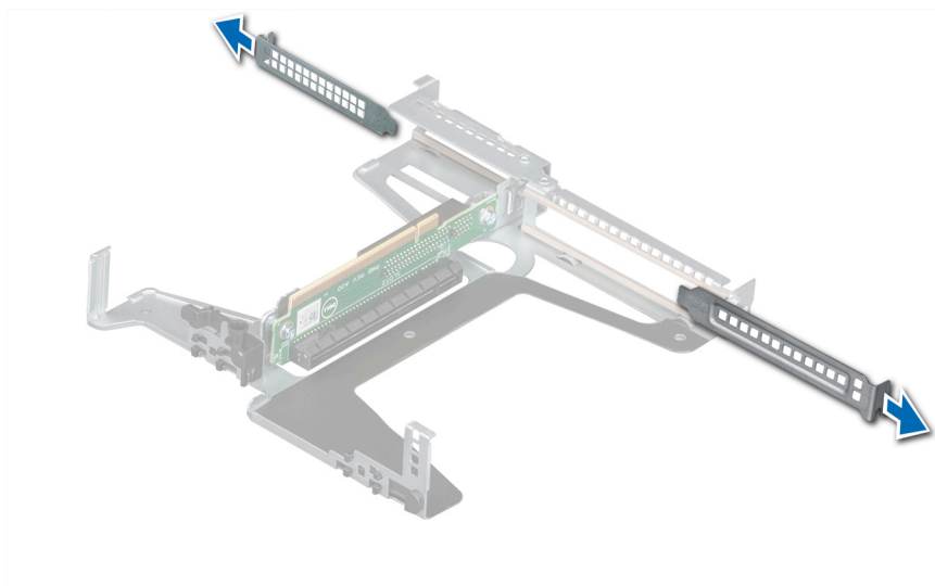
Figura 45. Extracción de la tarjeta de expansión de relleno
