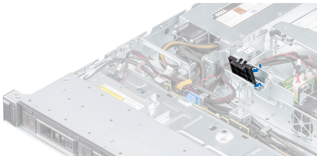
Figura 15. Extracción del ventilador de relleno
