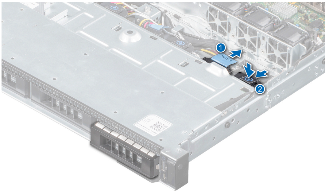
Figura 29. Extracción de una unidad cableada
