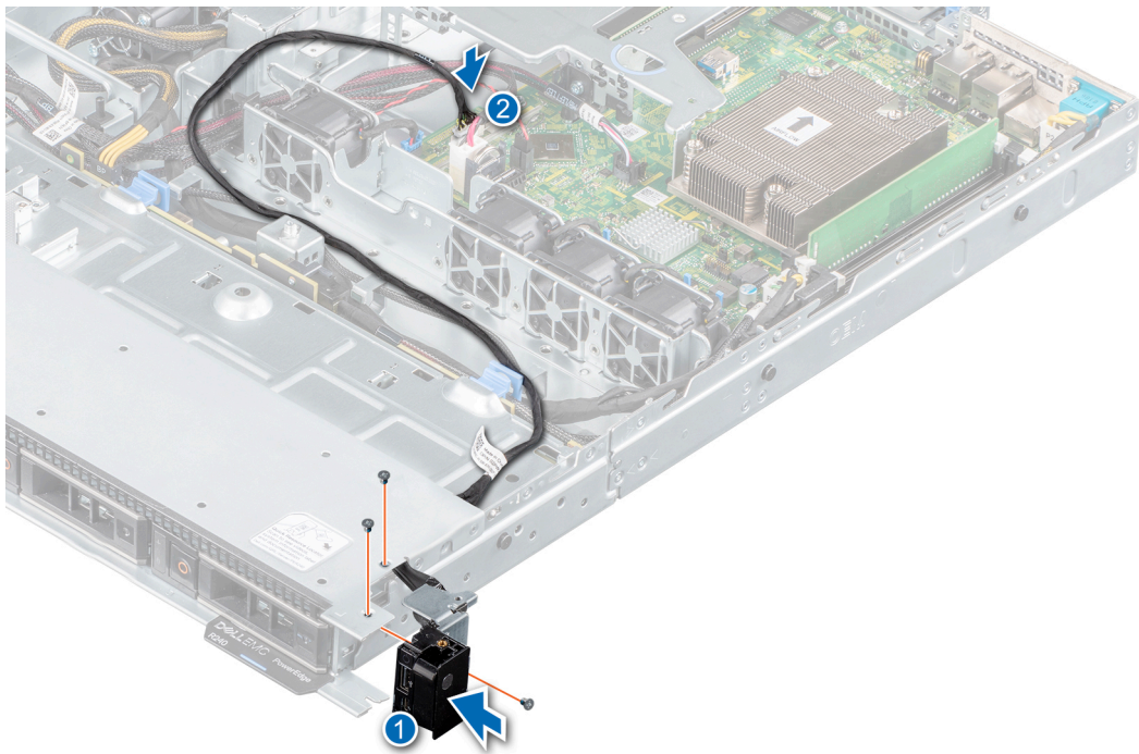
Figura 78. Instalación del panel de control derecho
