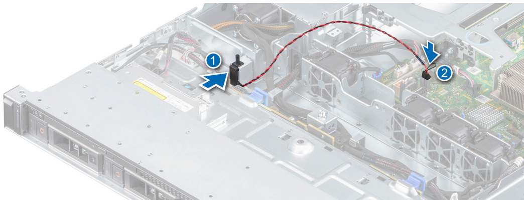
Figura 34. Instalación del interruptor de intrusiones
