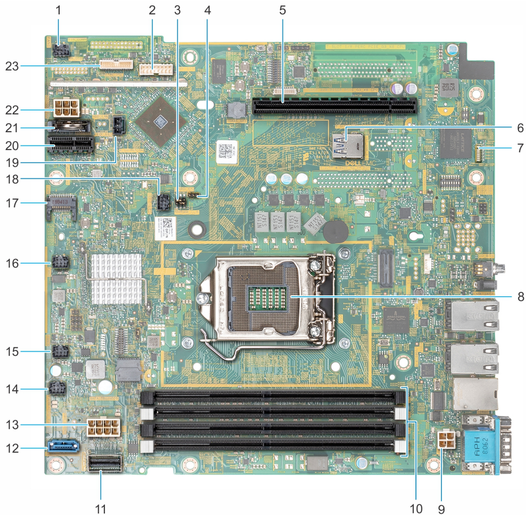
Figura 79. Conectores de la placa base
