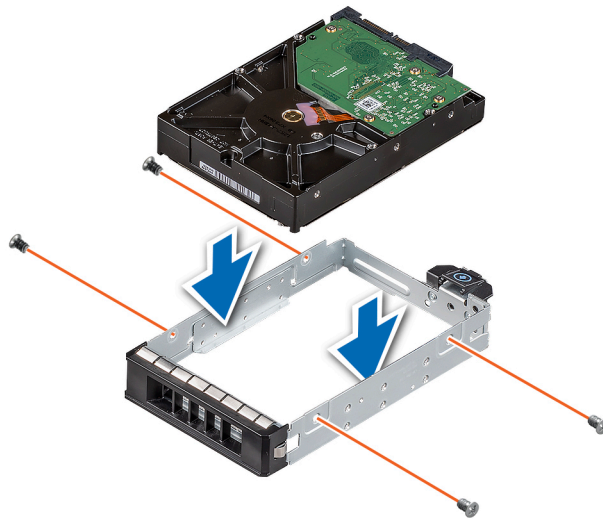
Figura 32. Instalación de una unidad cableada en el portauñidades
