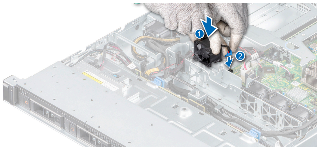
Figura 18. Instalación de un ventilador
