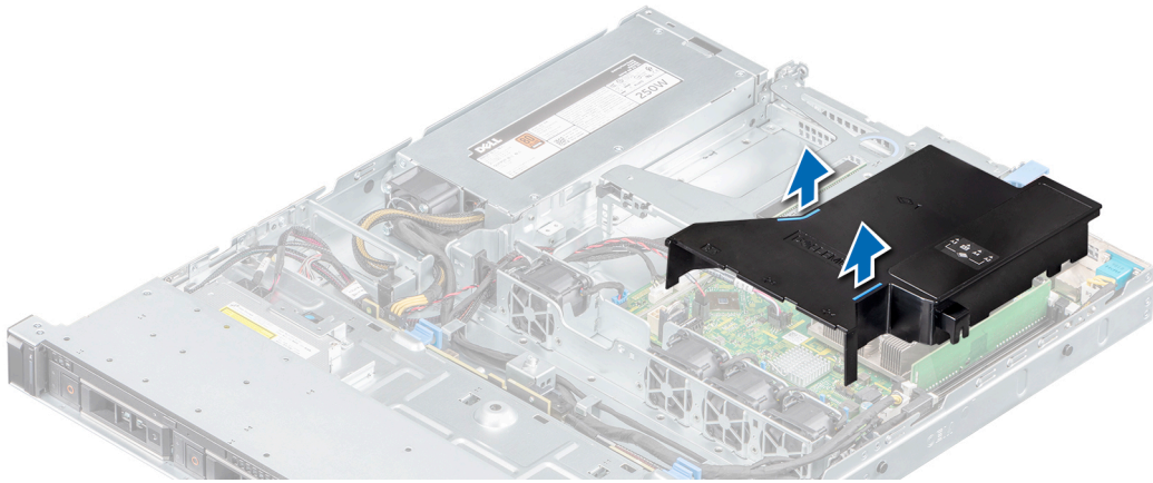
Figura 13. Extracción de la cubierta para flujo de aire
