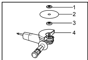
1. Contratuerca 2. Disco abrasivo de corte 3. Brida interior 4. Protector de disco para disco de corte
