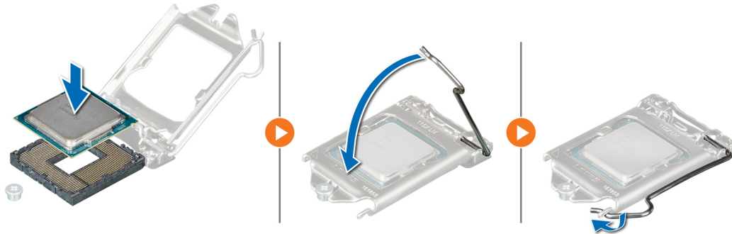
Ilustración 45. Instalación del procesador
