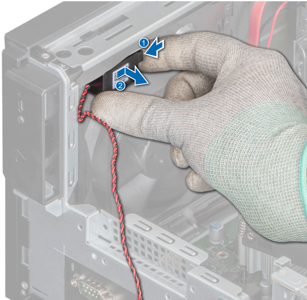
Ilustración 34. Extracción del altavoz
