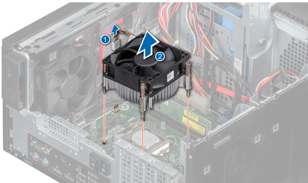
Ilustración 43. Extracción del disipador de calor
