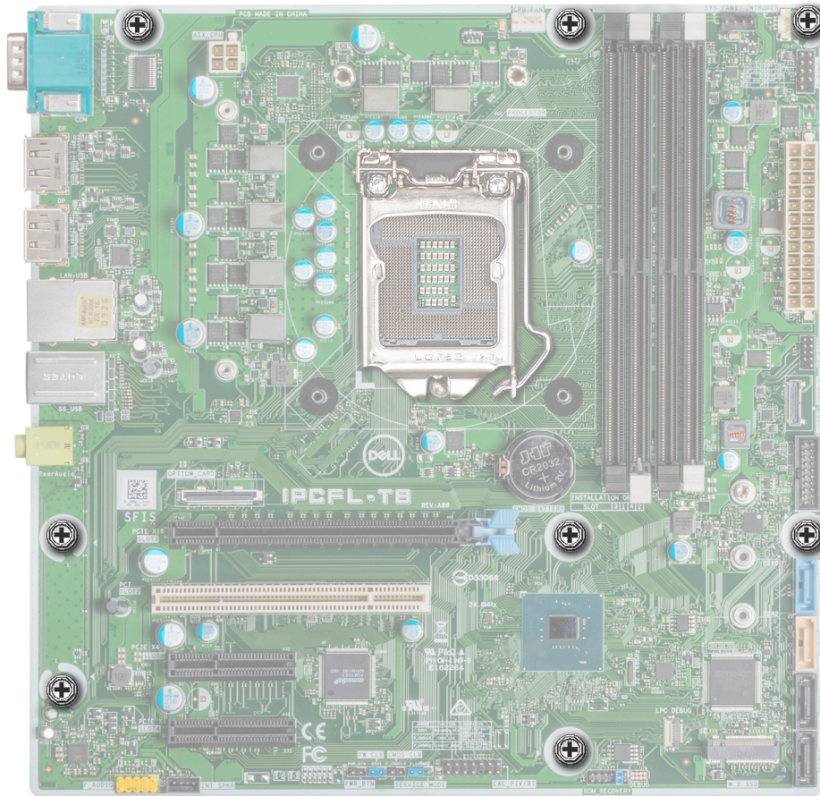
Ilustración 48. Ubicación de los tornillos de la placa base
