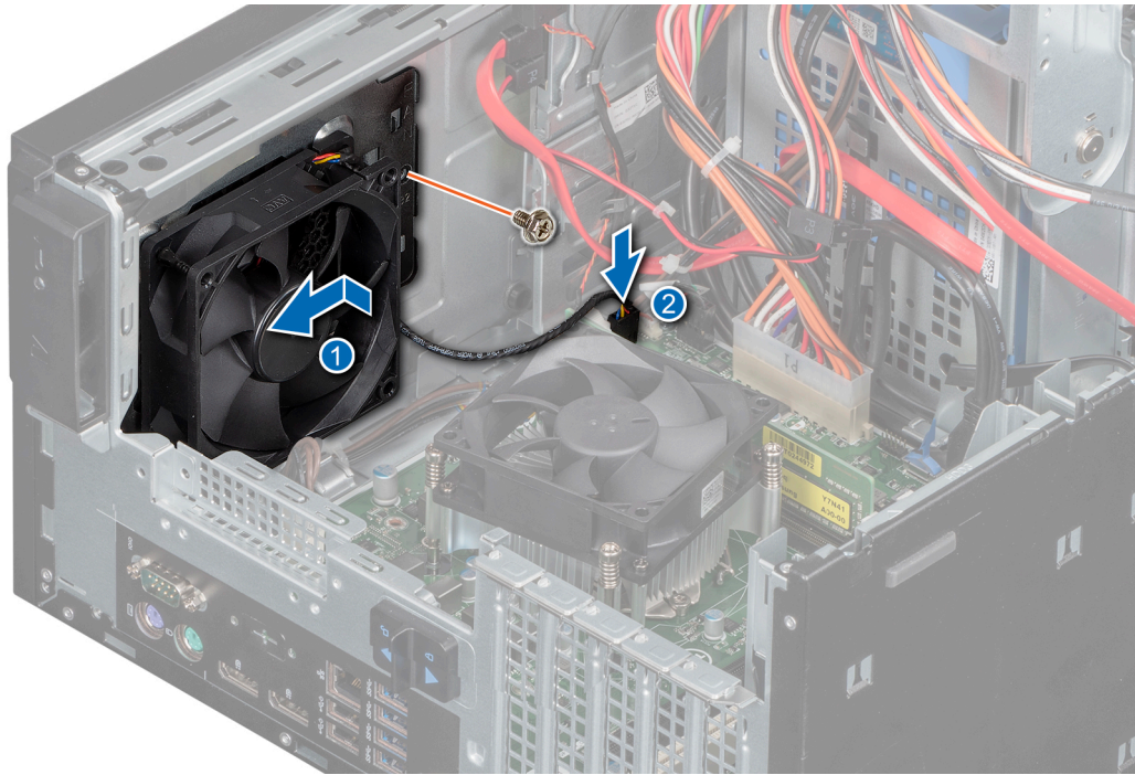
Ilustración 40. Instalación del soporte para el ventilador del sistema
