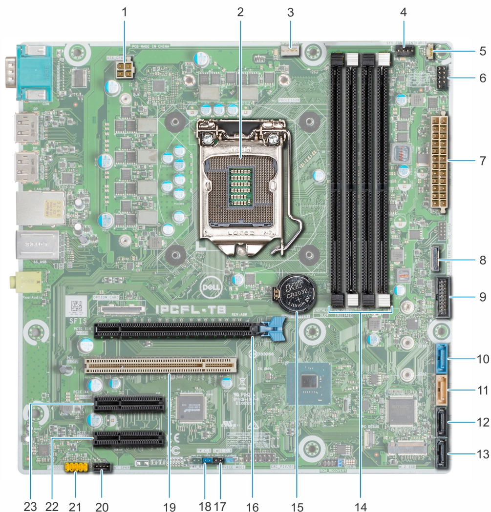
Ilustración 56. Puentes y conectores de la placa base
