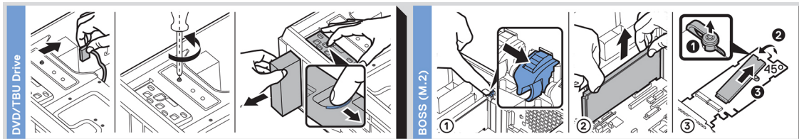
Figura 11. Instalación de DVD y BOSS
