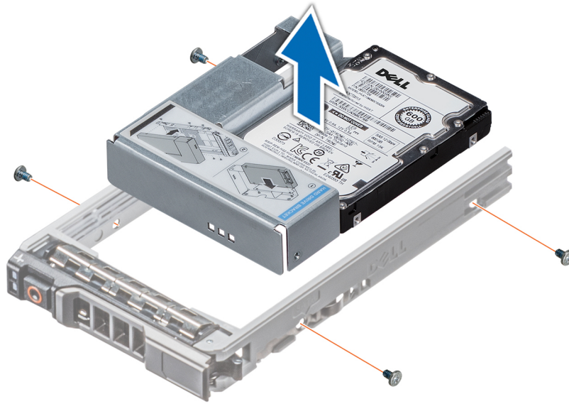
Figura 36. Extracción de un adaptador de unidad de 3.5 pulgadas de un portaunderidades de 3.5 pulgadas
