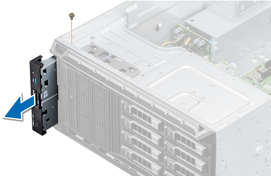
Figura 84. Extracción del ensamblaje del panel de control
