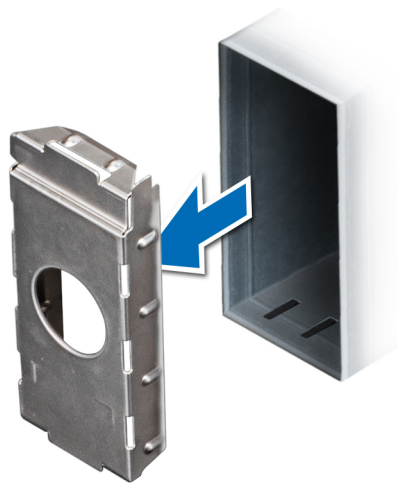
Figura 70. Extracción de la unidad de fuente de alimentación de relleno (PSU)
