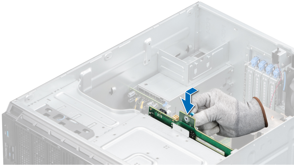
Figura 46. Instalación del backplane de la unidad
