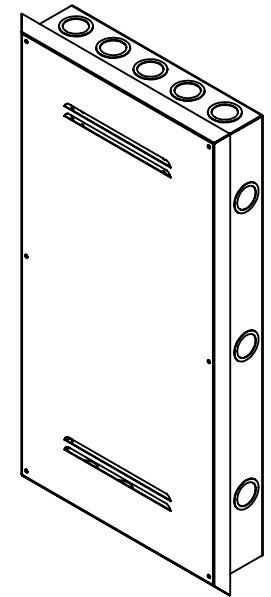
Gabinete EIGTR28 con Accesorio EIGTR28C (No incluido)
