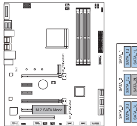
1x M.2 SATA SSD Slot -- 5x SATA HDDs
