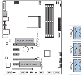
2x M.2 SATA SSD Slot -- 5x SATA HDDs
