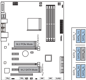
1x M.2 PCIe SSD Slot + 1x M.2 SATA SSD Slot -- 5x SATA HDDs
