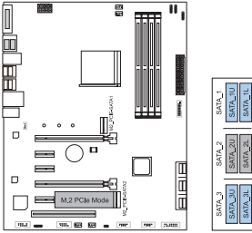
1x M.2 PCIe SSD Slot -- 4x SATA HDDs
