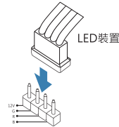
RGB LED裝置接頭 (12V_LED)
