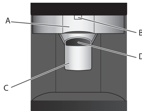
A. Paleta del despachador de agua C. Paleta del despachador de hielo B. Pico del despachador de agua D. Guía para el hielo
