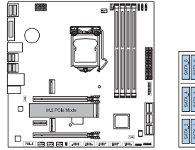
1x N/A + 1x M.2 PCIe SSD Slot -- 6x SATA HDDs
