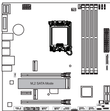
1x N/A + 1x М.2 SATA SSD Slot -- 3x SATA HDDs
