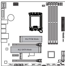
1x М.2 SATA SSD Slot + 1x М.2 PCIe SSD Slot -- 3x SATA HDDs
