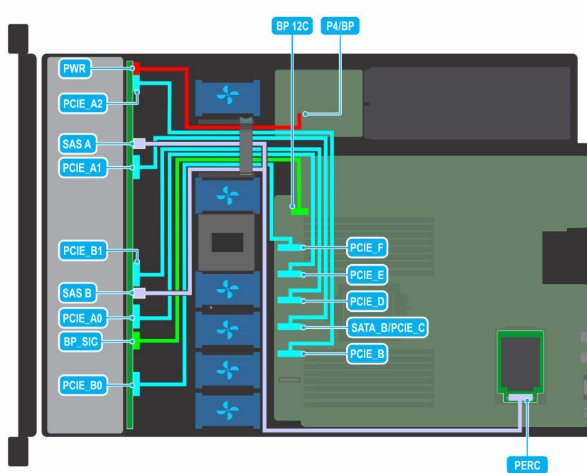
Ilustración 41. Enrutamiento de cables: backplane de unidad de 10 x 2,5 pulgadas a la controladora integrada (NVMe)
