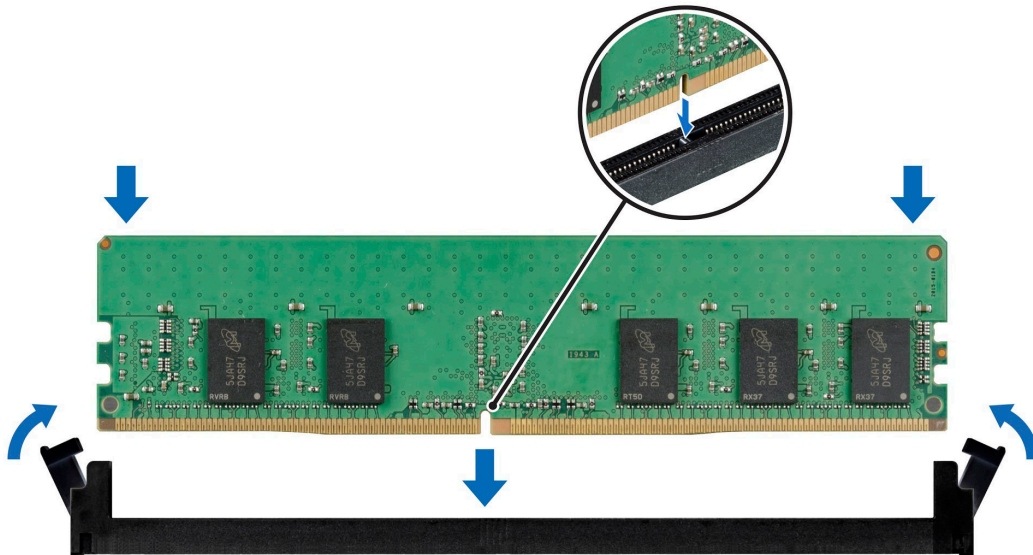
Ilustración 44. Instalación de un módulo de memoria
