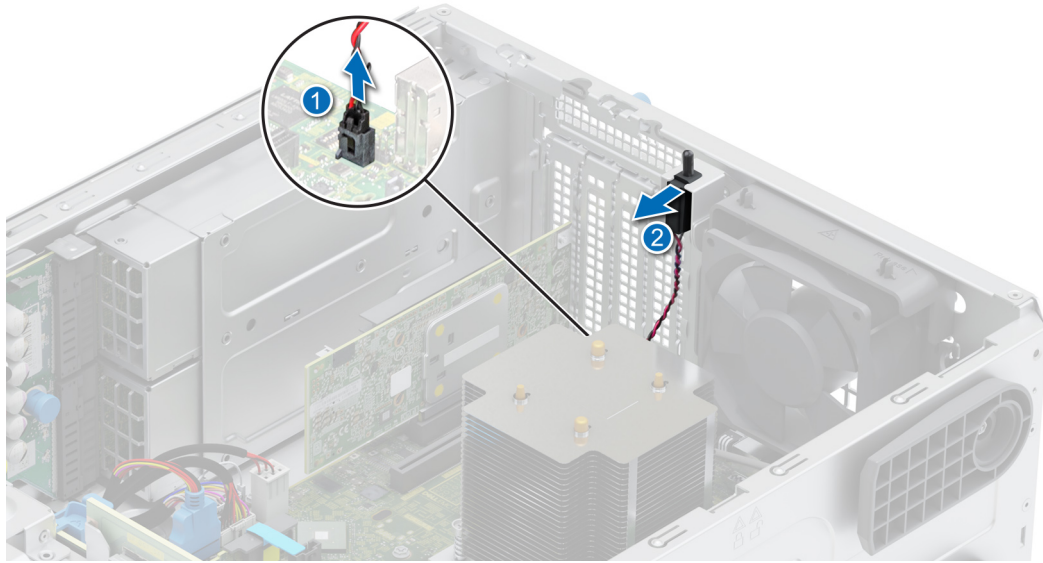
Ilustración 20. Extracción del módulo del interruptor de intrusiones
