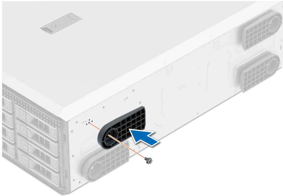
Ilustración 15. Instalación de los pies del sistema
