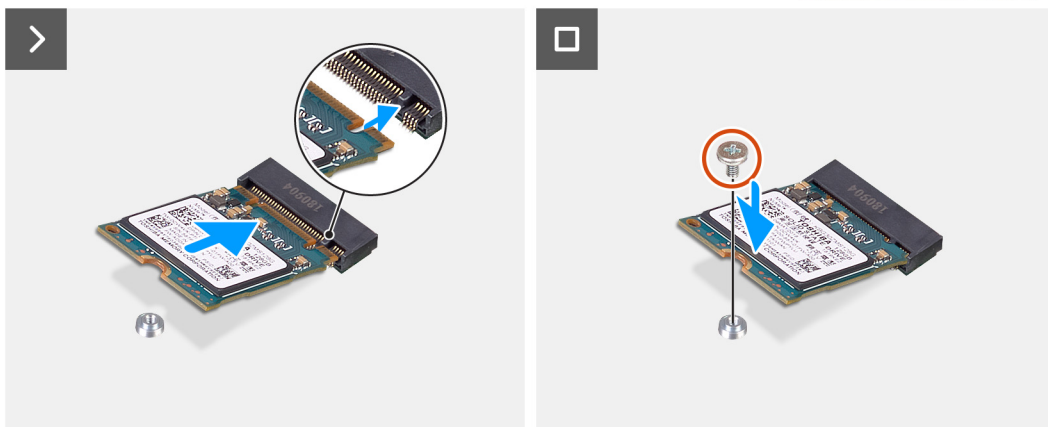
Ilustración 24. Instalación de la unidad de estado sólido M.2 2230 en la ranura 1
