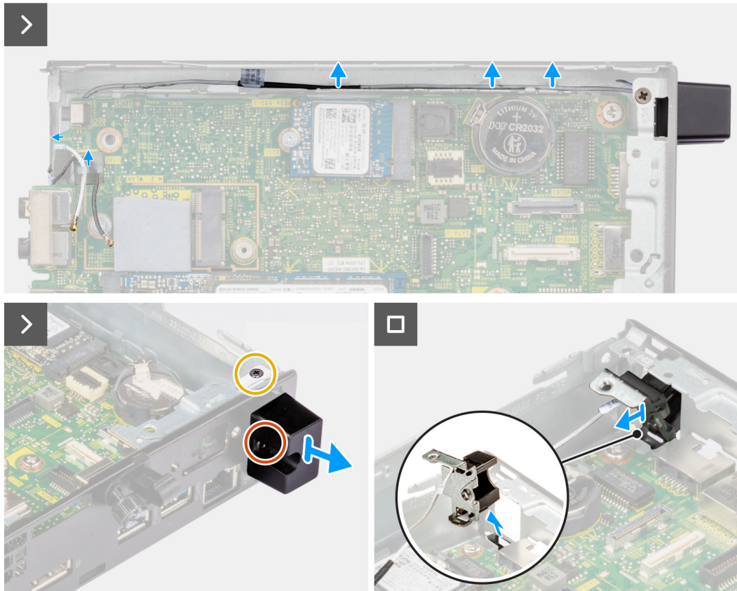
Ilustración 50. Extracción del módulo de la antena (cable blanco)
