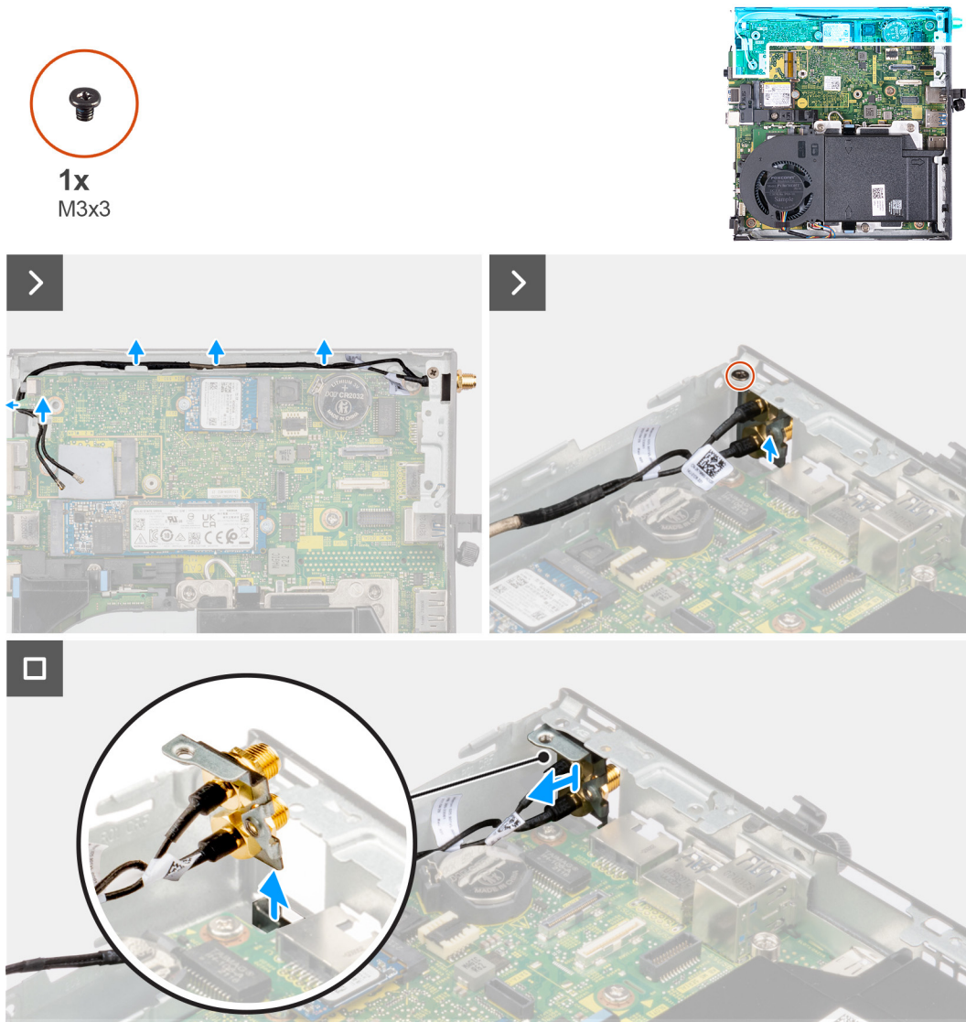
Ilustración 54. Extracción de la antena de SMA (ubicación 3)
