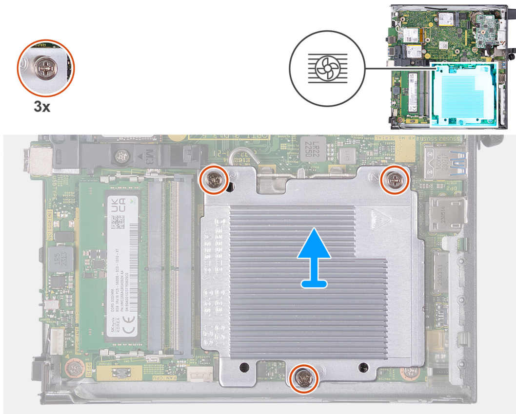
Ilustración 40. Extracción del disipador de calor
