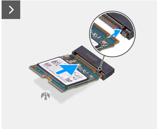
Ilustración 20. Instalación de la unidad de estado sólido 2230 en la ranura 0
