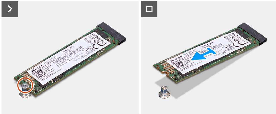
Ilustración 19. Extracción de la unidad de estado sólido M.2 2280
