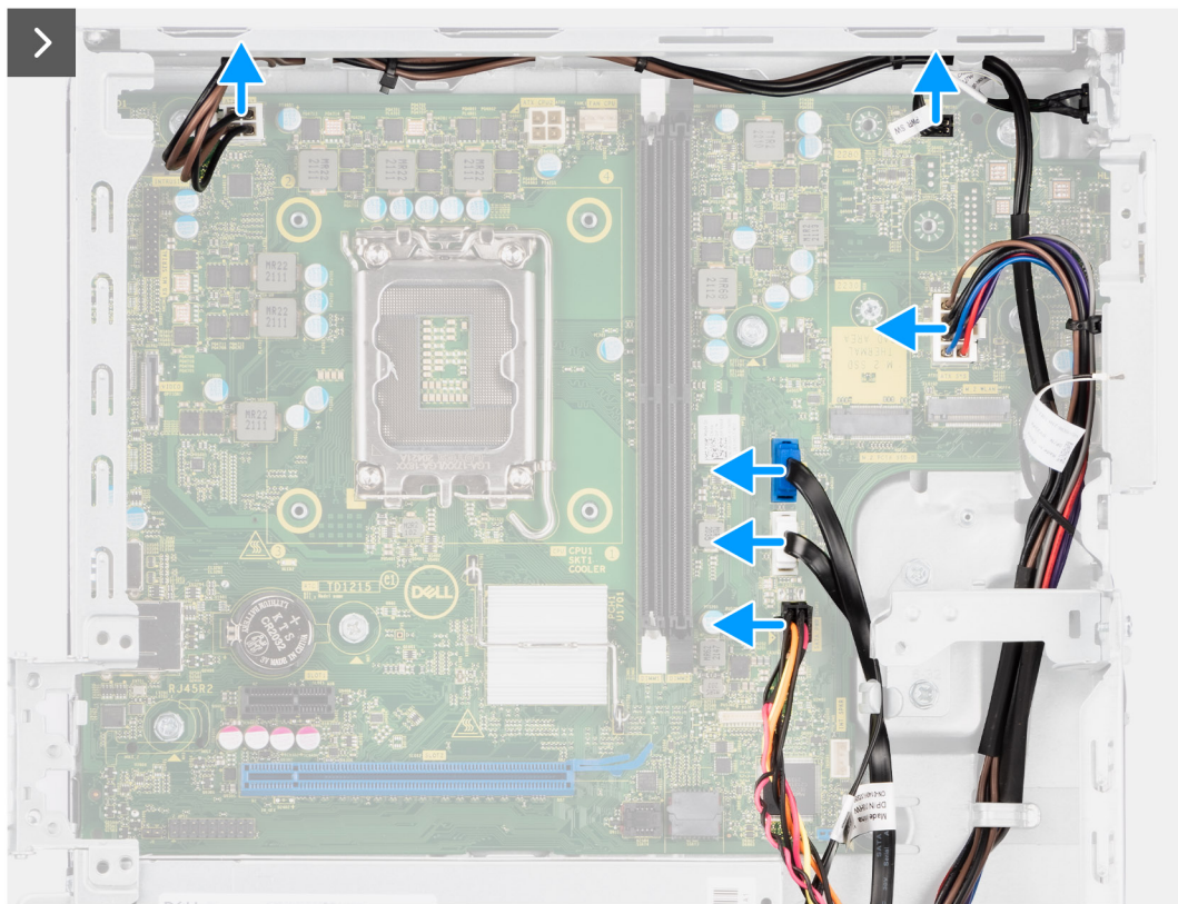
Ilustración 58. Extracción de la tarjeta madre
