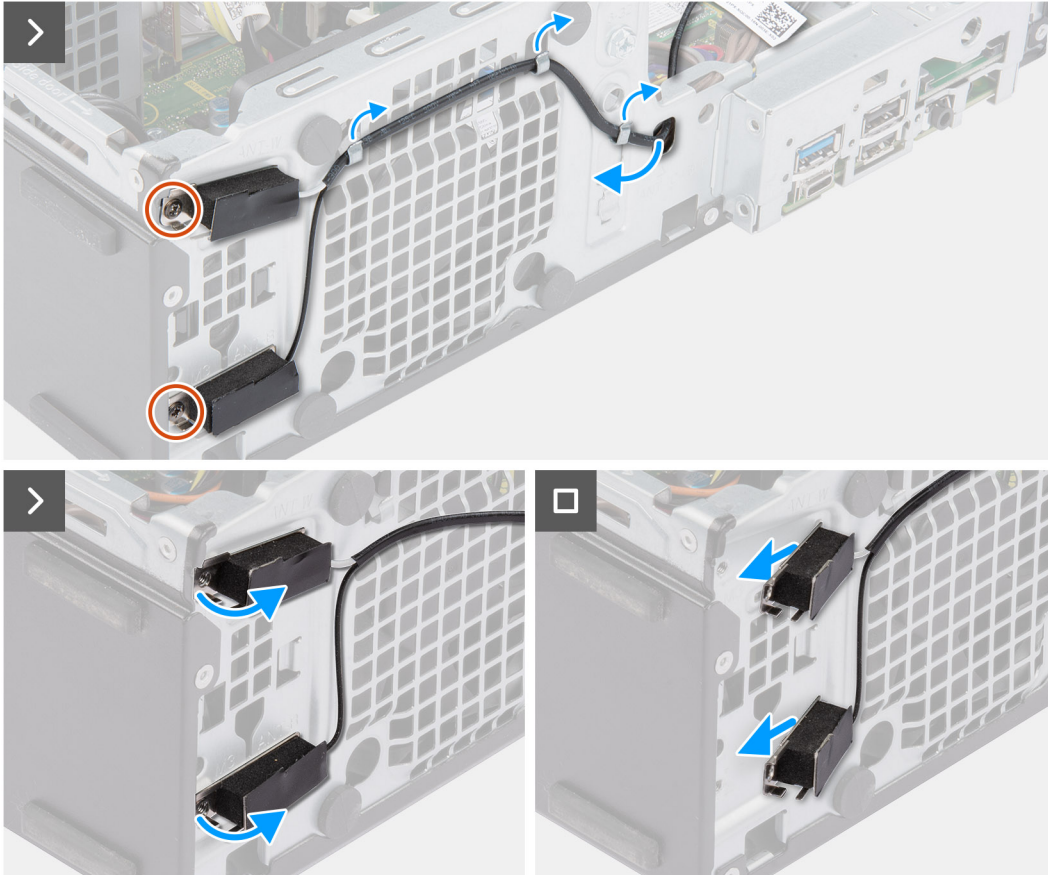
Ilustración 37. Extracción del módulo de la antena interna
