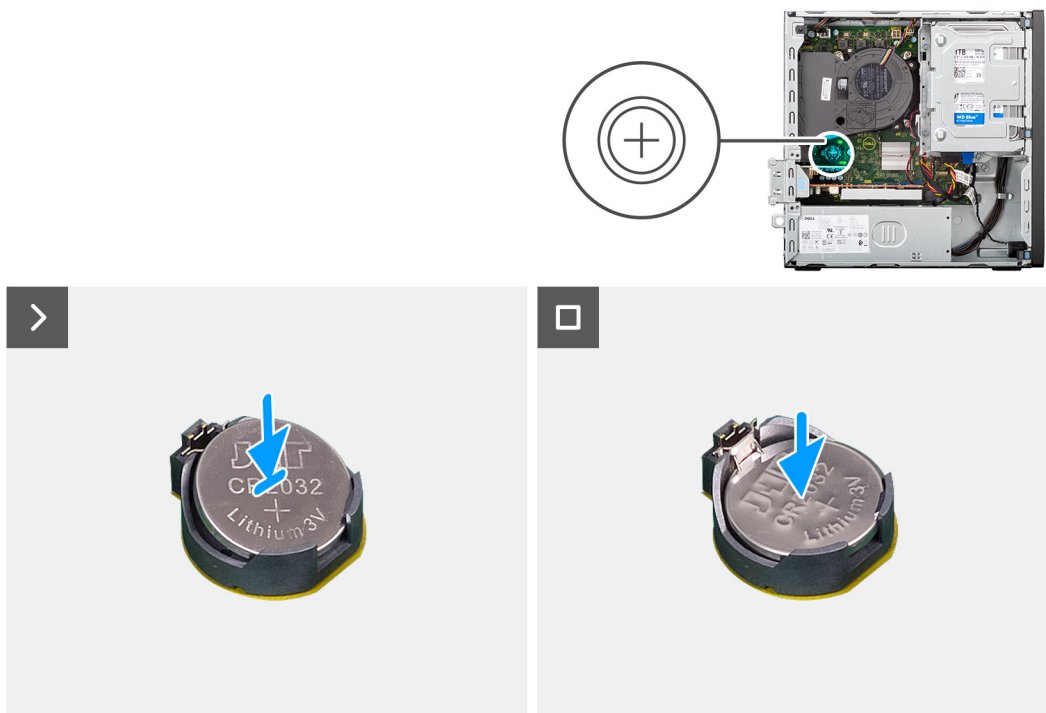
Ilustración 6. Instalación de la batería de tipo botón
