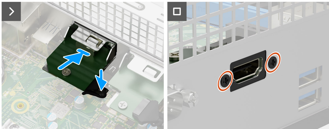
Ilustración 55. Instalación del módulo de HDMI
