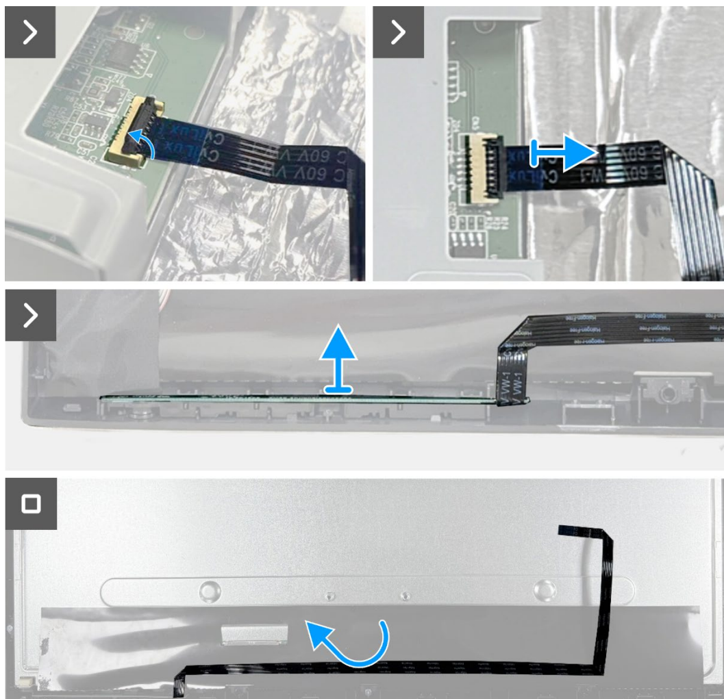
Figura 15. Retire la placa del teclado
