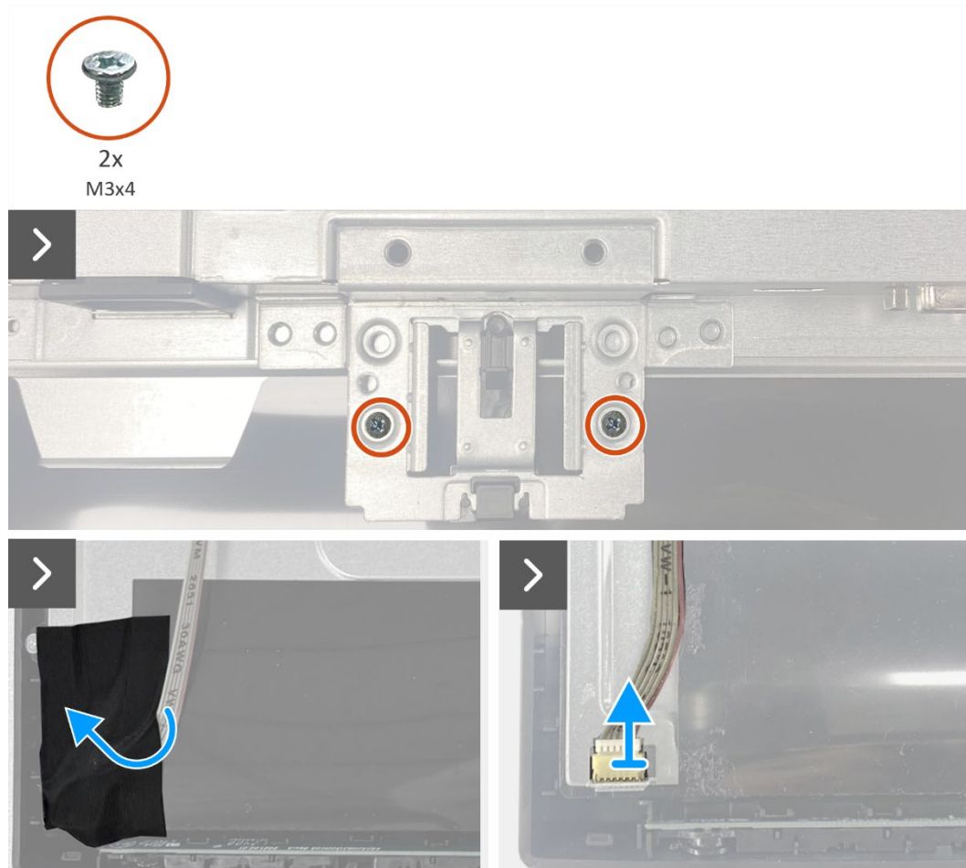
Figura 17. Retirar el conjunto del chasis
