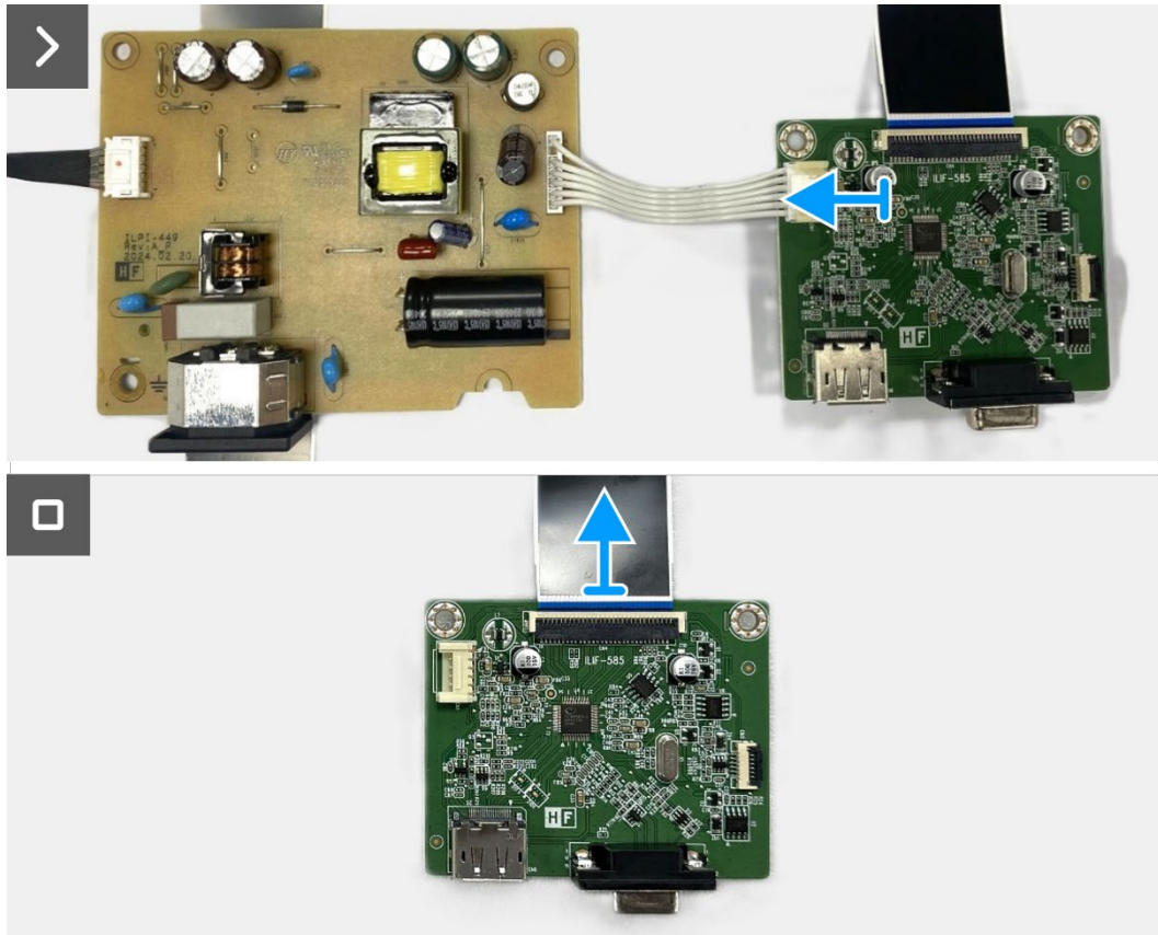
Figura 22. Retire la placa de la interfaz
