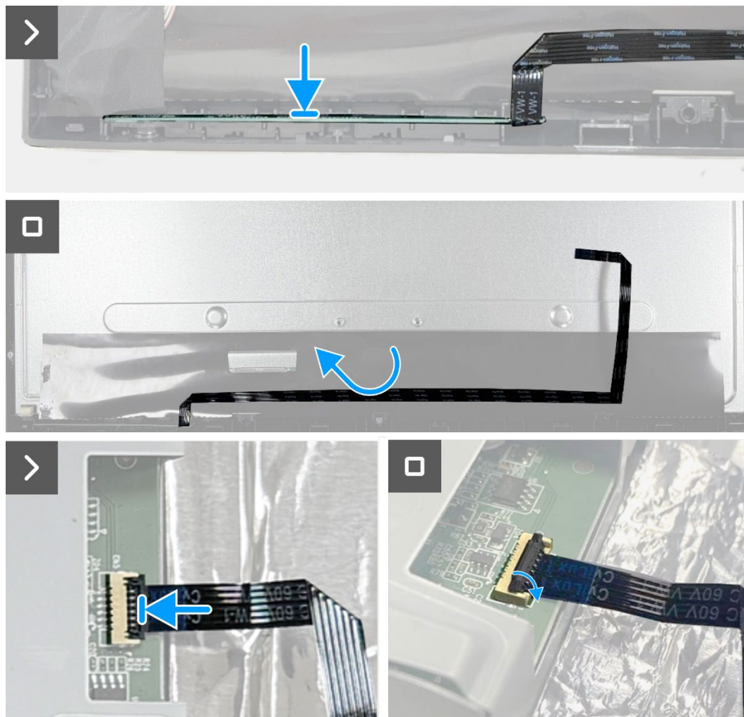
Figura 16. Instalar la placa del teclado
