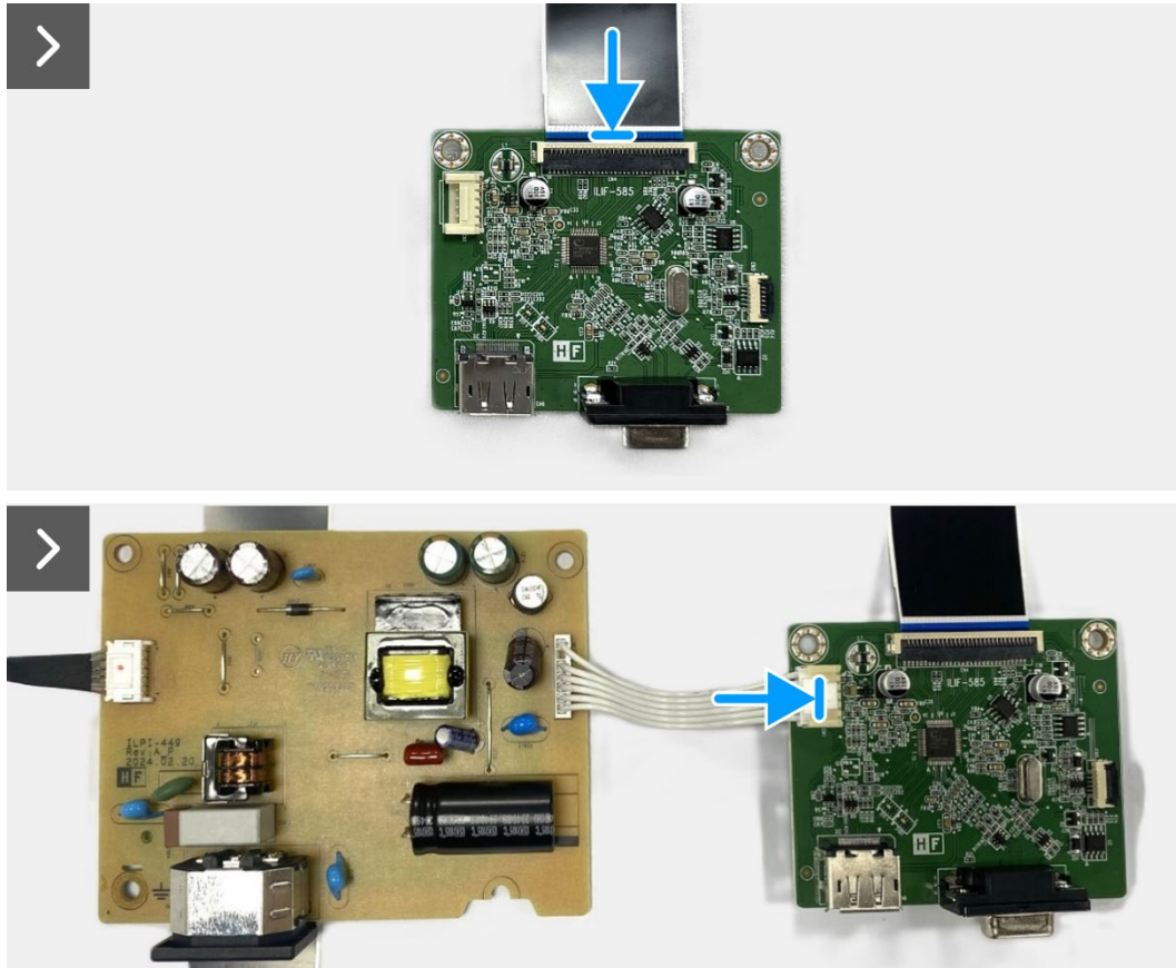
Figura 23. Instalar la placa de la interfaz
