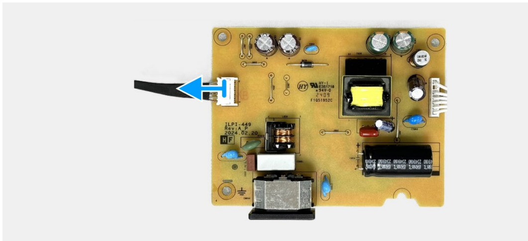
Figura 25. Retire la placa de alimentación
