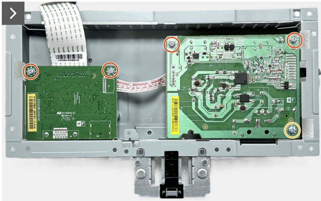
Figura 21. Retire la placa de la interfaz
