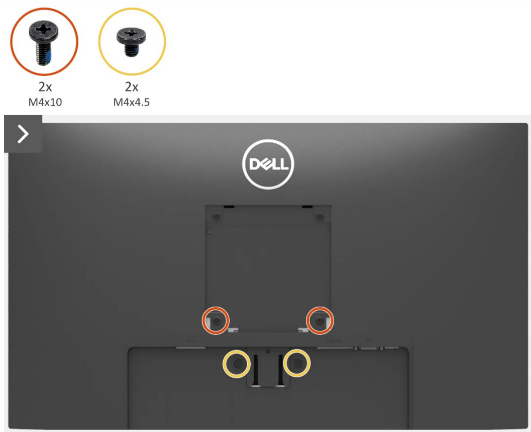
Figura 12. Quitar el cubierta posterior
