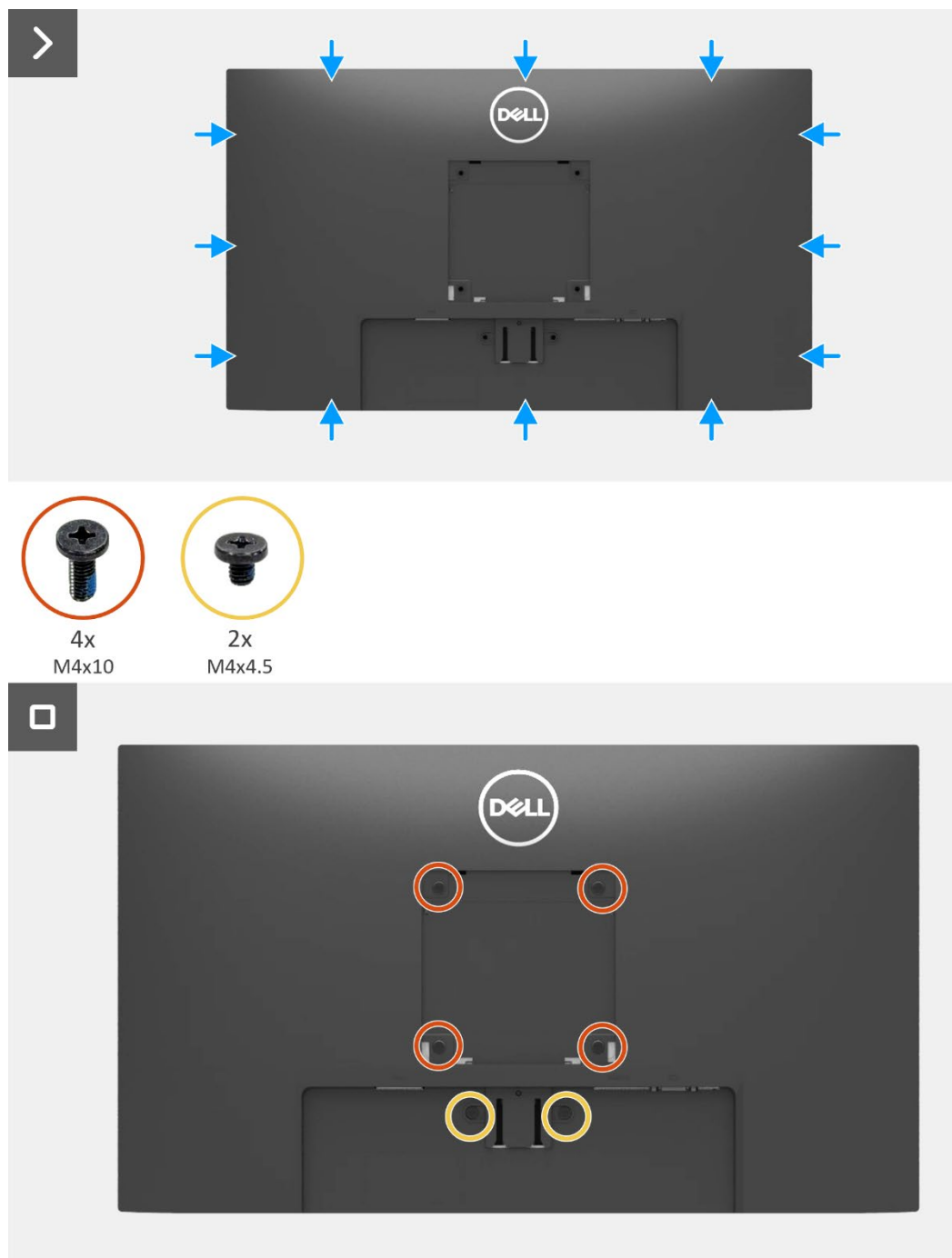
Figura 14. Instalar la cubierta posterior
