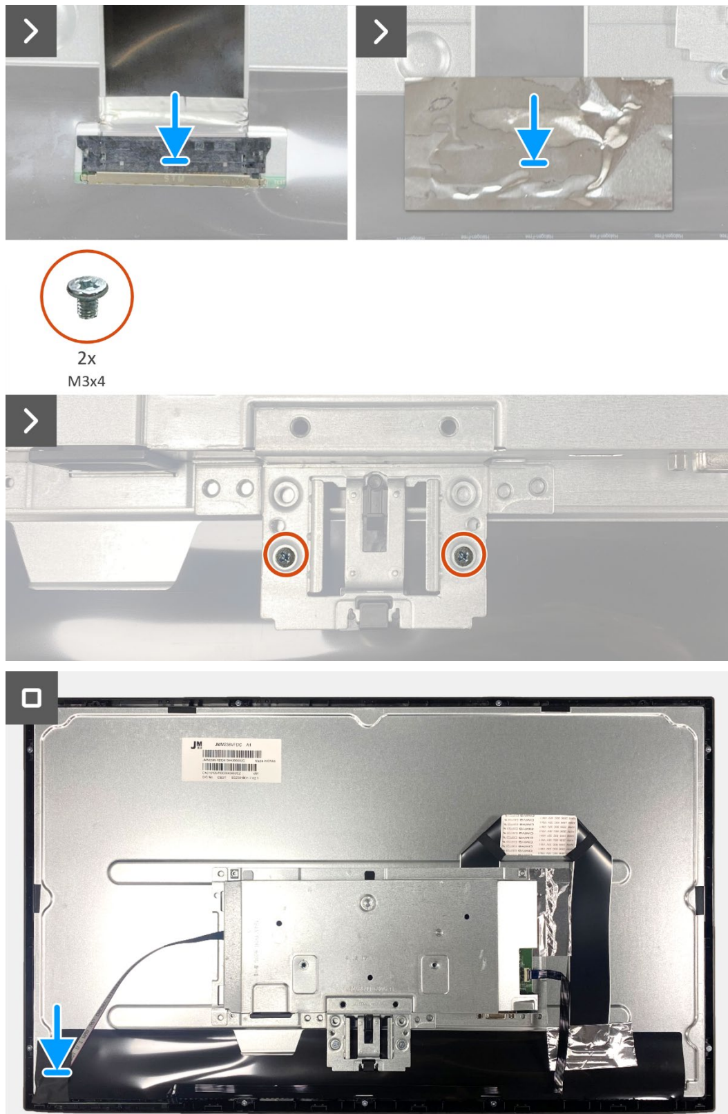
Figura 19. Instalar el conjunto del chasis
