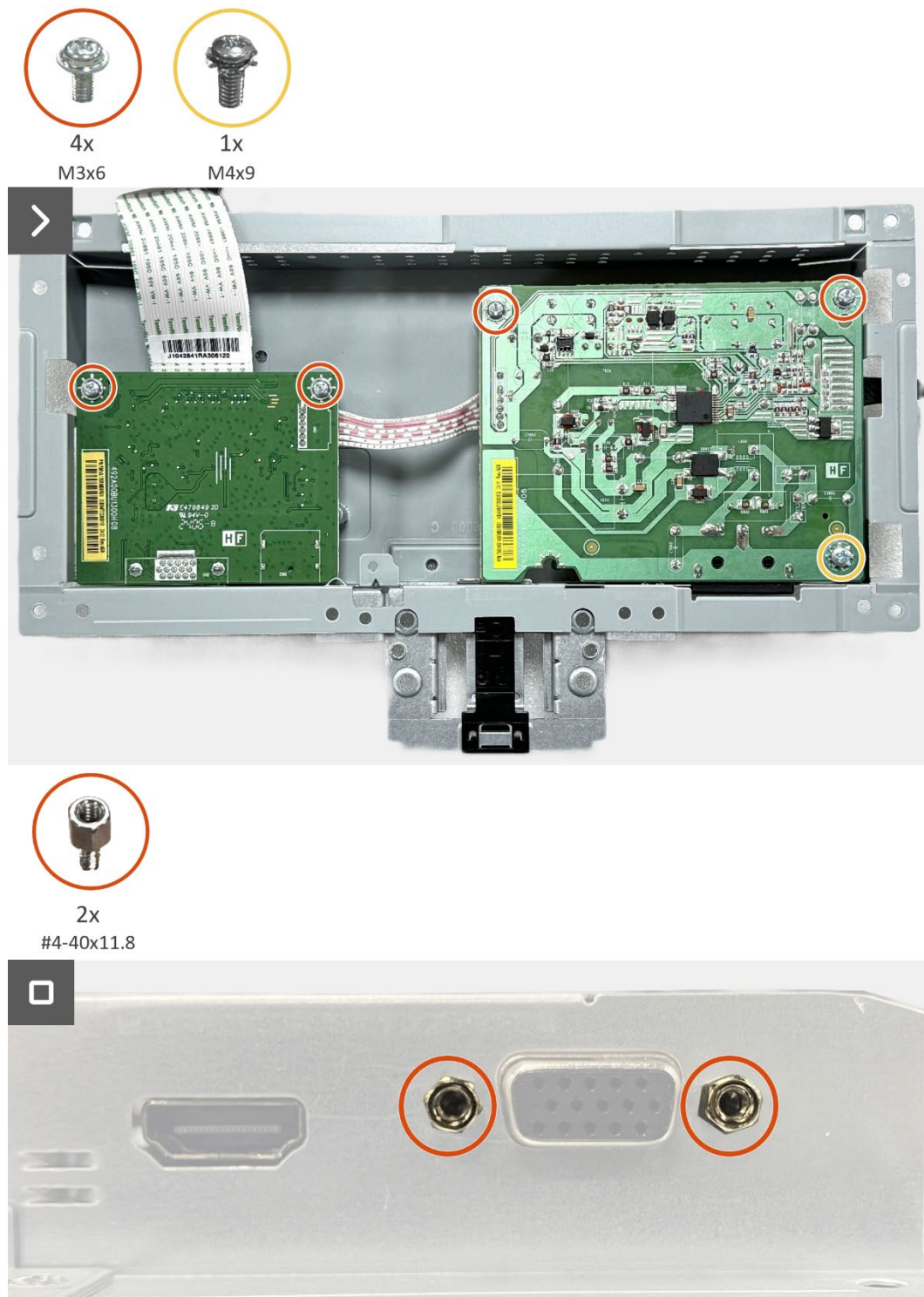
Figura 24. Instalar la placa de la interfaz
