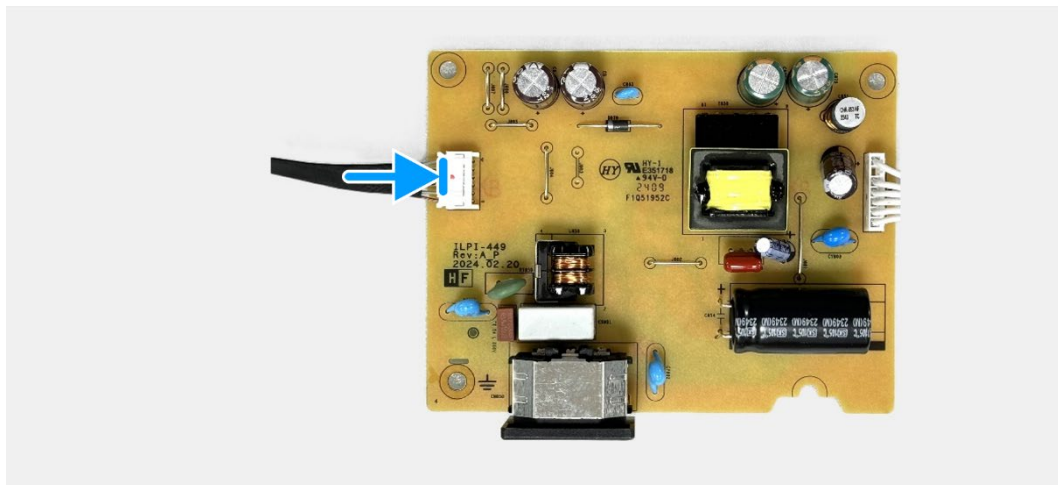
Figura 26. Instalar la placa de alimentación
