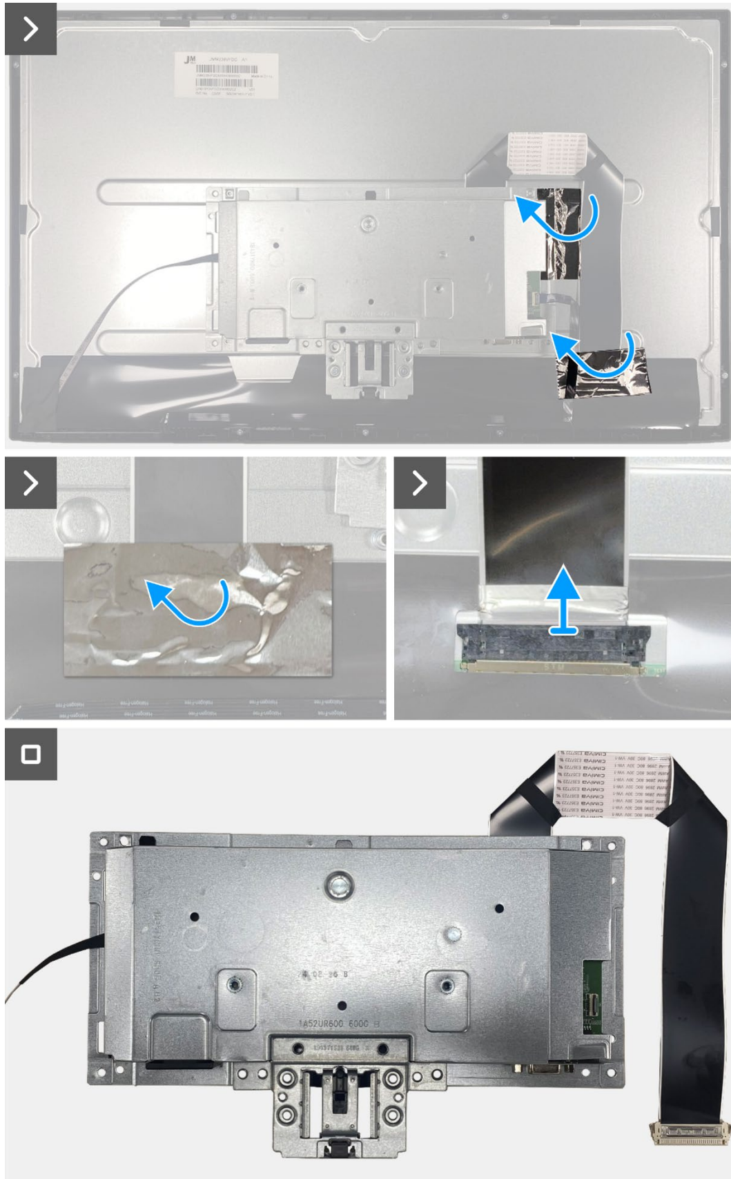
Figura 18. Retirar el conjunto del chasis
