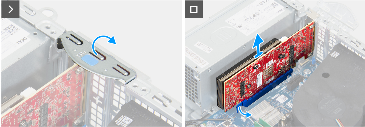
Ilustración 27. Extracción de la tarjeta gráfica
