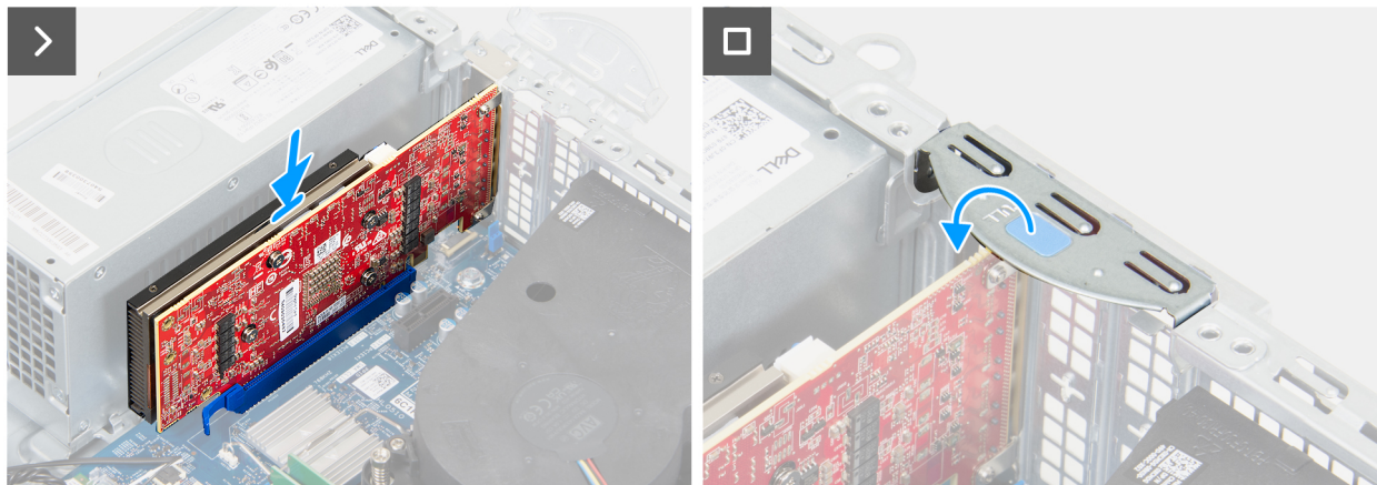
Ilustración 28. Instalación de la tarjeta gráfica
