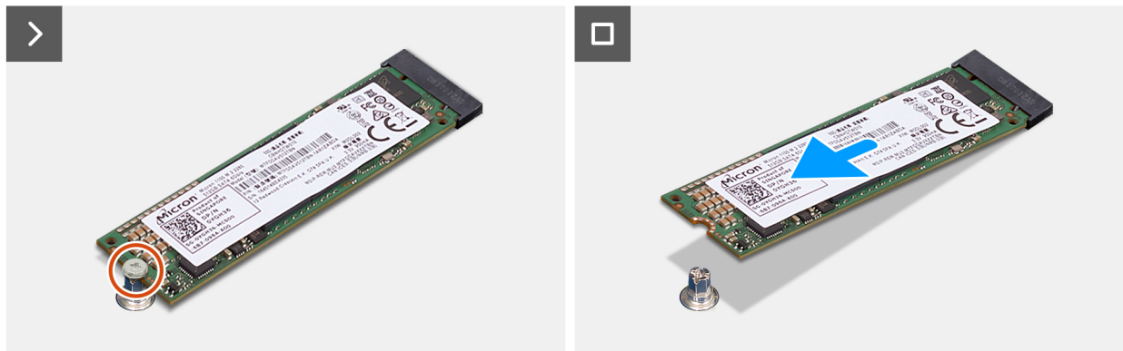
Ilustración 24. Extracción de la unidad de estado sólido M.2 2280
