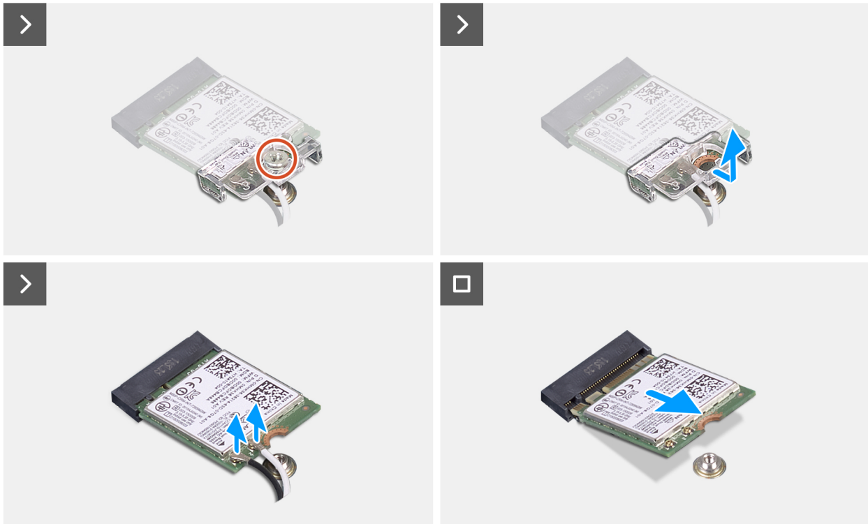
Ilustración 29. Extracción de la tarjeta inalámbrica
