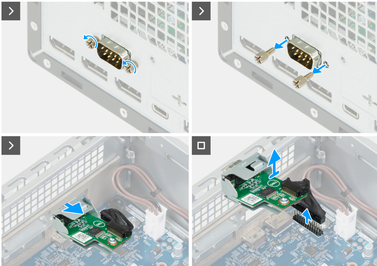
Ilustración 57. Extracción del módulo de puerto serial
