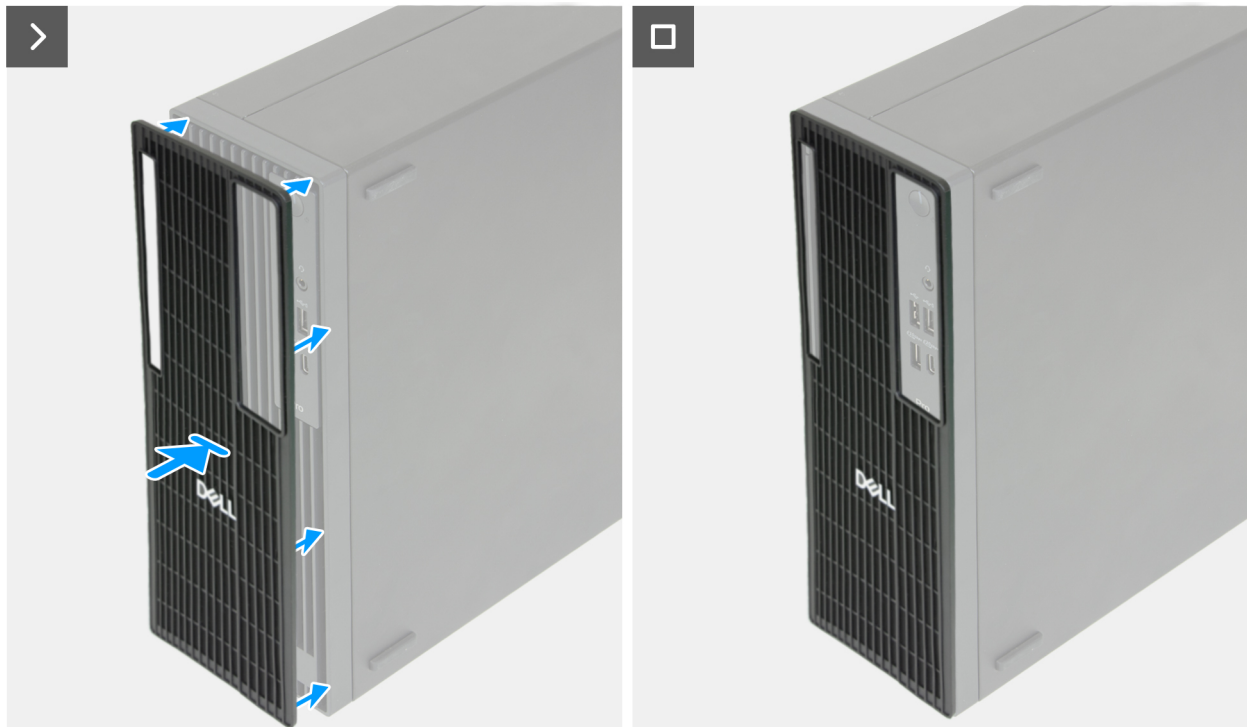
Ilustración 15. Cómo instalar el filtro antipolvo
