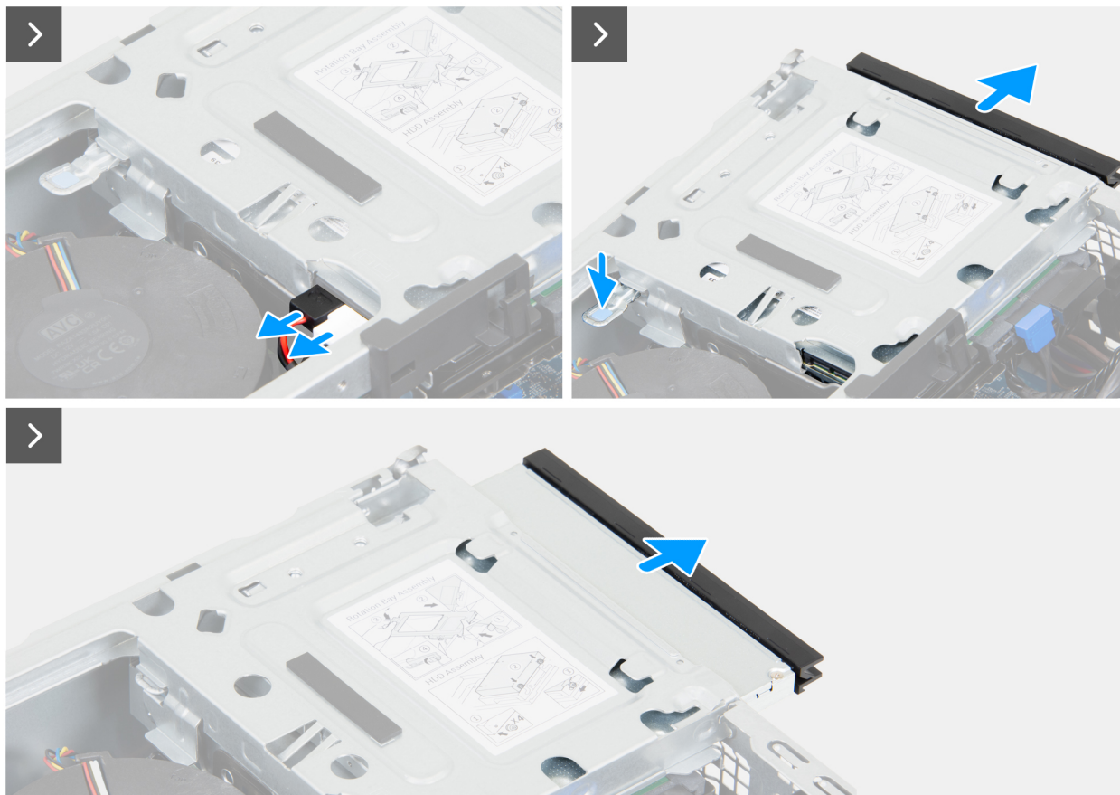
Ilustración 31. Extracción de la unidad óptica
