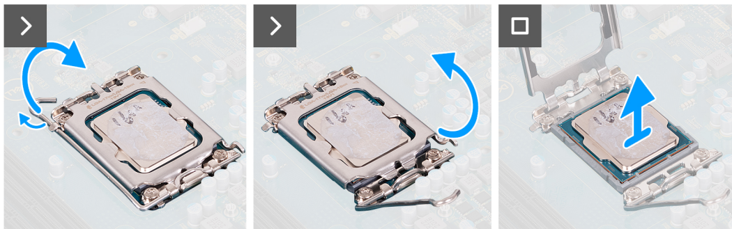
Ilustración 60. Extracción del procesador
