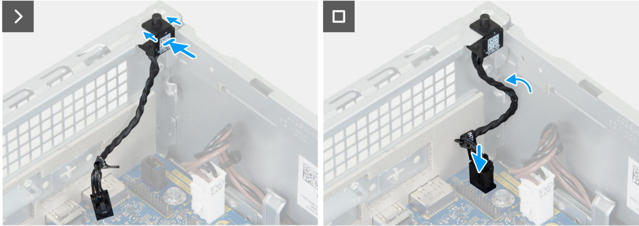
Ilustración 43. Instalación del switch de intrusión
