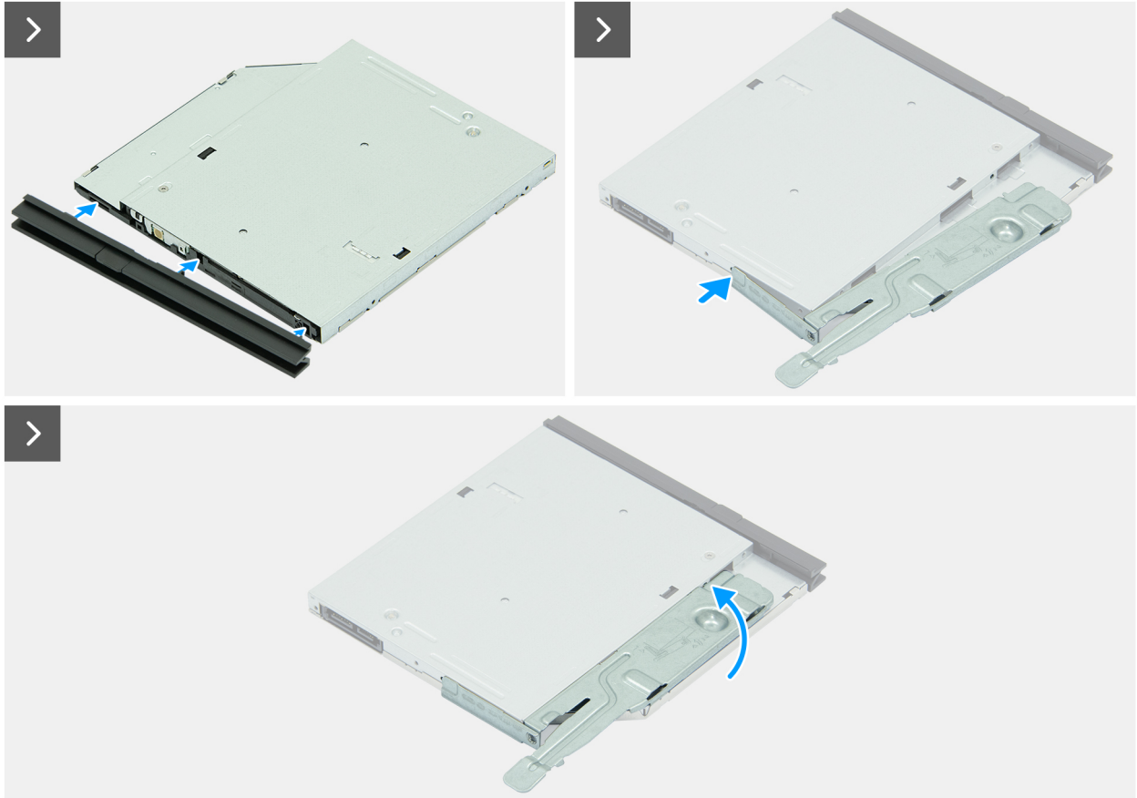
Ilustración 33. Instalación de la unidad óptica
