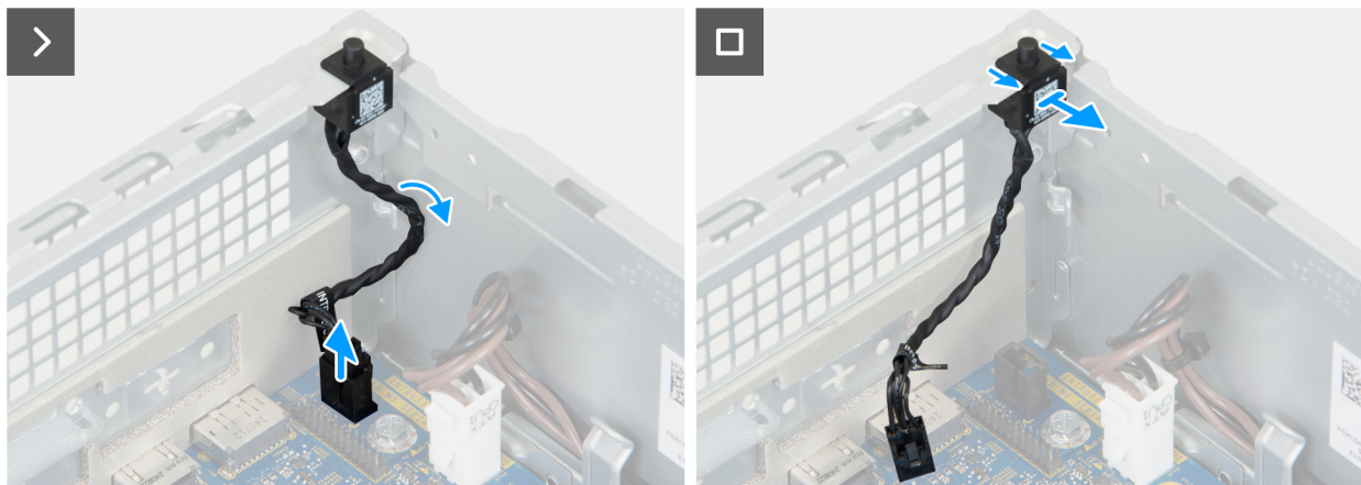
Ilustración 42. Extracción del switch de intrusiones
