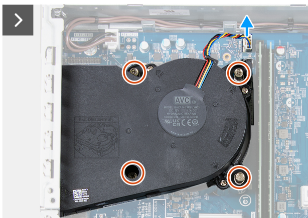
Ilustración 52. Extracción del ensamblaje del disipador de calor y el ventilador del procesador
