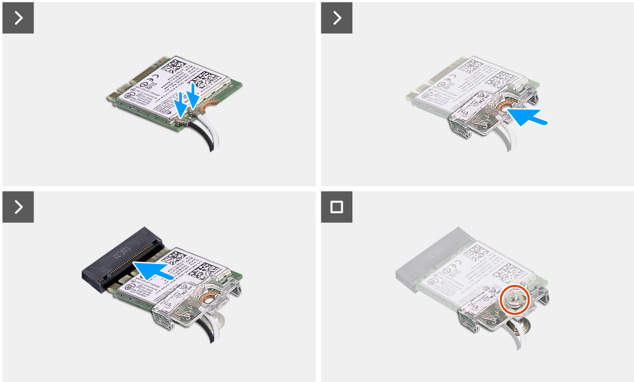
Ilustración 30. Instalación de la tarjeta inalámbrica
