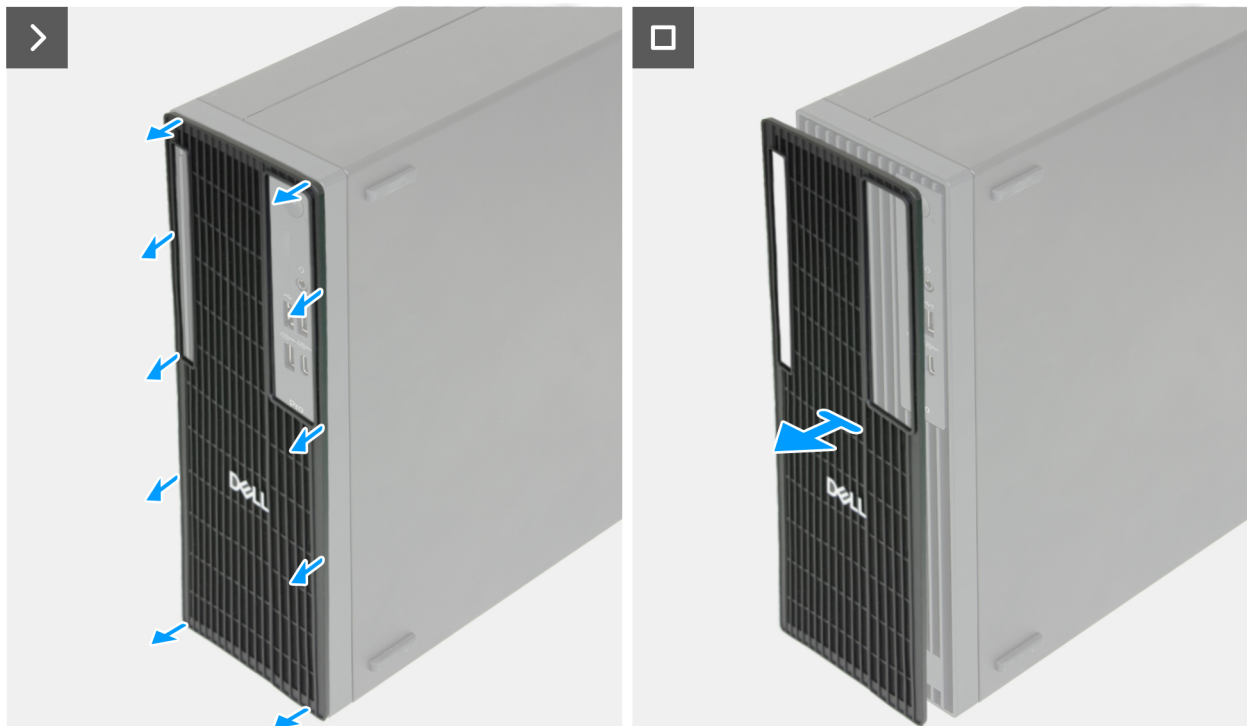
Ilustración 14. Extracción del filtro antipolvo
