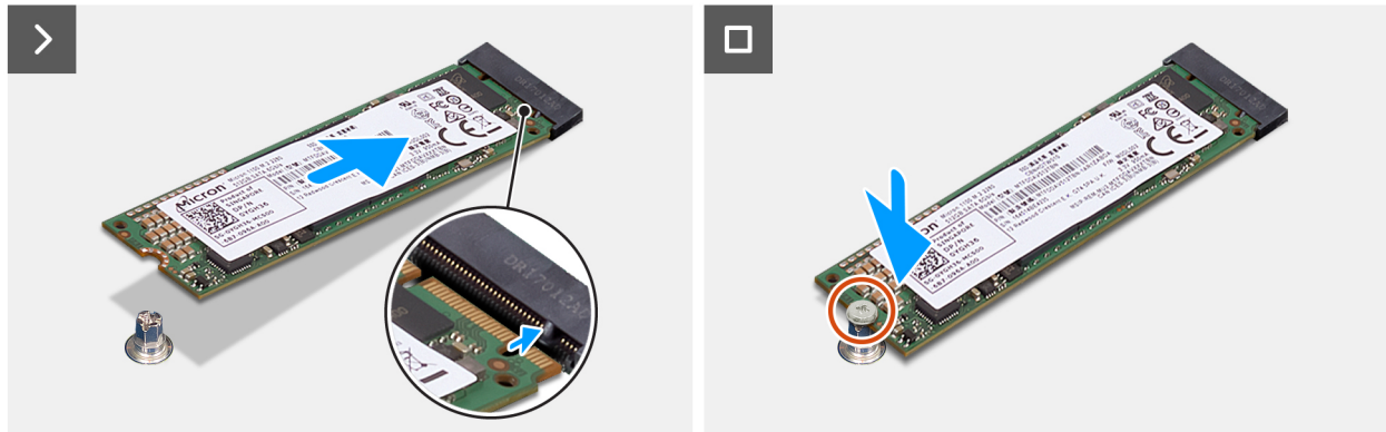
Ilustración 25. Instalación de la unidad de estado sólido M.2 2280
