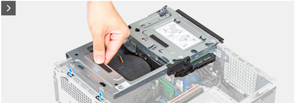
Ilustración 35. Extracción de la bahía de unidad
