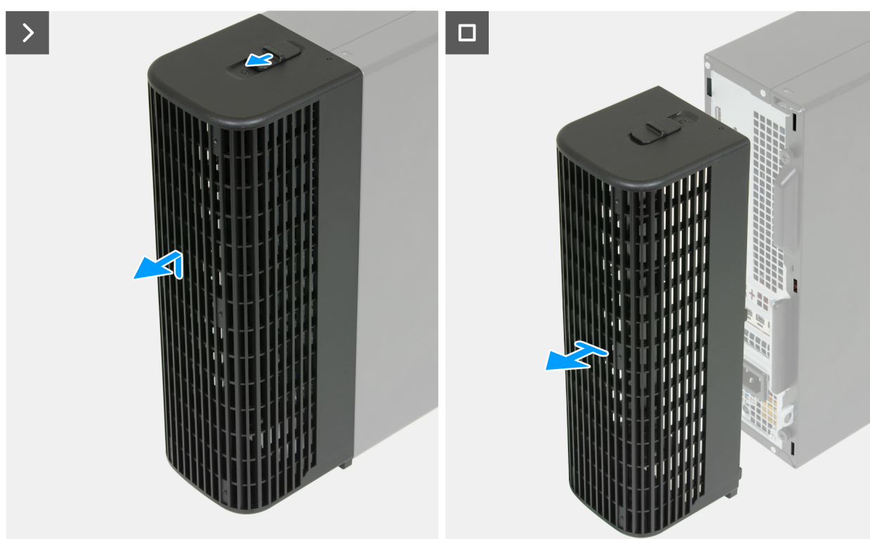
Ilustración 4. Extracción de la cubierta de cables
