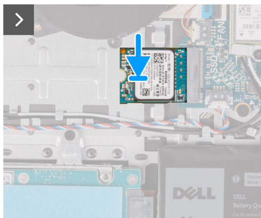
Ilustración 7. Instalación de la unidad de estado sólido
