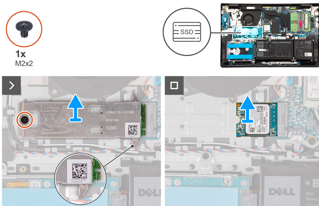
Ilustración 6. Extracción de la unidad de estado sólido
