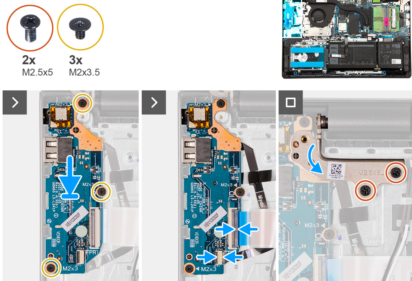
Ilustración 8. Instalación de la placa secundaria de I/O
