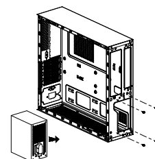
8. Instalación de la fuente de alimentación 8. PSU install
