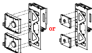
6. Combina la posición para 1*SSD o 1*HDD 6. Combine 1*SSD or 1*HDD position
