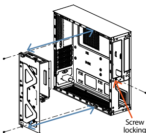
4. Posición de la unidad óptica (bloqueo con tornillo) 4. Position of optical drive (Screw locking)
