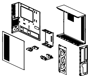
1. Estructura de los componentes del gabinete 1. Decomposition diagram of case structure
