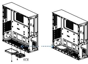
5. Posición opcional para la unidad SSD y (ventilador 6 cm) 5. SSD and 6cm fan position optional
