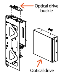
7. Desatornillar la instalación de la unidad óptica (Sujeción de la unidad óptica, Unidad de lectura óptica) 7. Unscrew optical drive install (Optical drive buckle, Optical drive)
